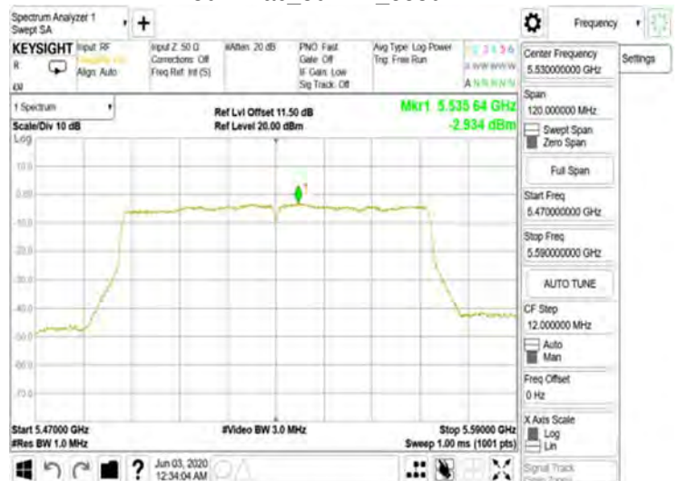
802.11ac 80MHz 5530MHz
