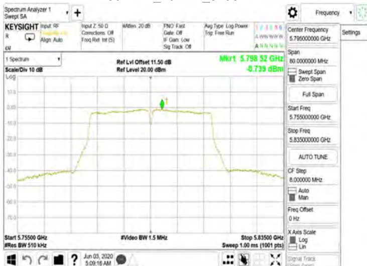
802.11n 40MHz 5795MHz
