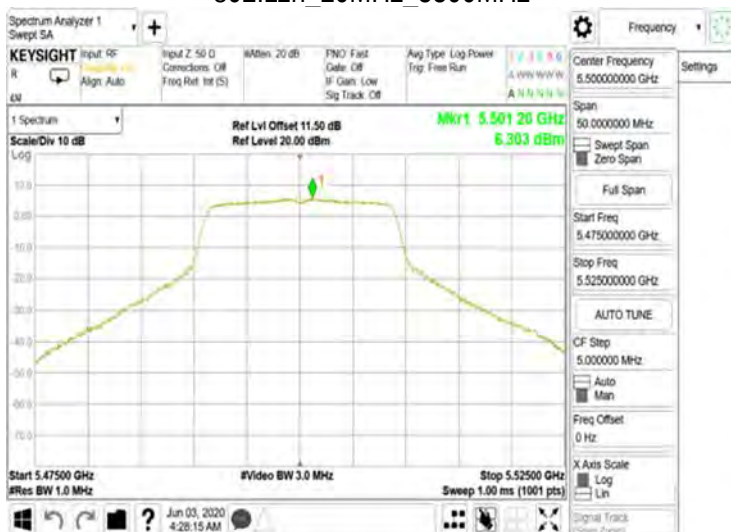
802.11n_20MHz_5500MHz
