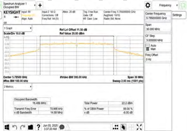
FCC 802.11a 20MHz Chain0 5785MHz
