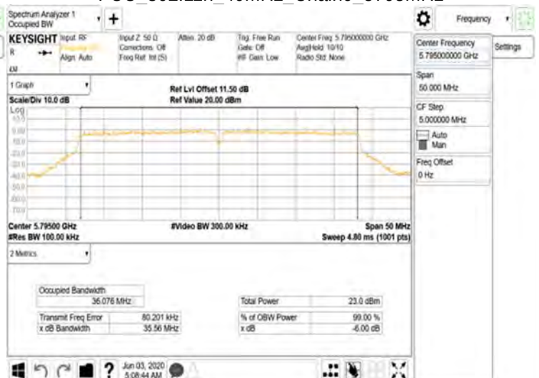
FCC 802.11n_40MHz_Chain0_5795MHz
