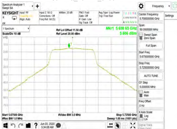
802.11a_20MHz_5700MHz
