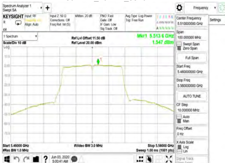
802.11n_40MHz_5510MHz
