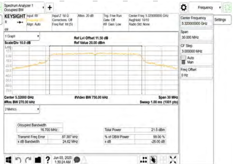
FCC 802.11a 20MHz Chain0 5320MHz
