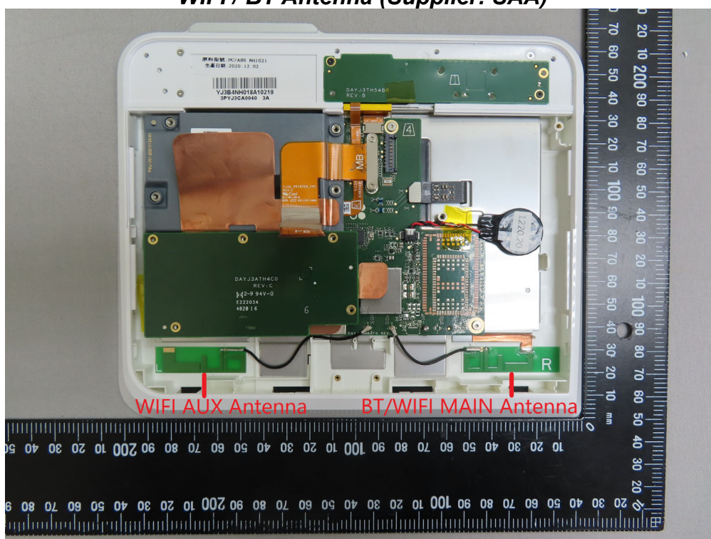
WIFI / BT Antenna (Supplier: SAA)
