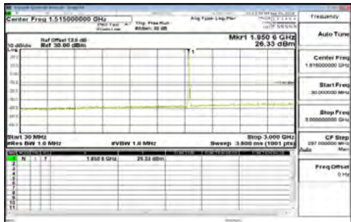
30MHz~3GHz_Band2_10MHz_QPSK_1_0_LowCH18650-1855
