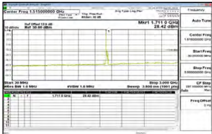
30MHz~3GHz_Band4_20MHz_QPSK_1_0_LowCH20050-1720
