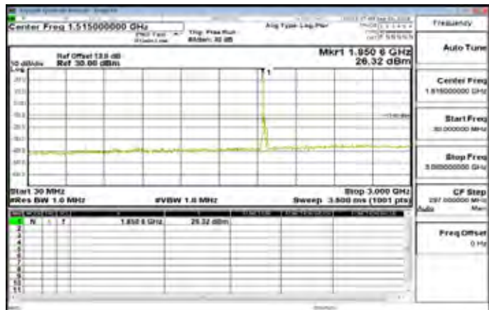
30MHz-3GHz_Band2_20MHz_QPSK_1_0_LowCH18700
