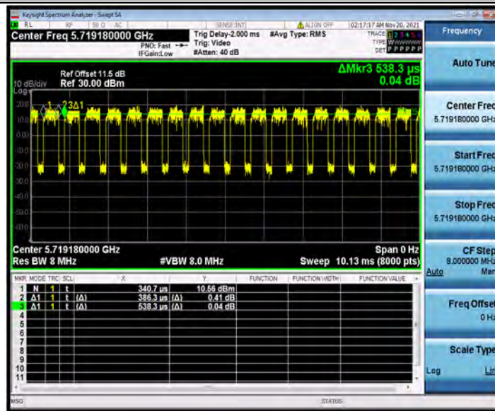
11AX20MIMO_Ant1_5720_26Tone_RU8
