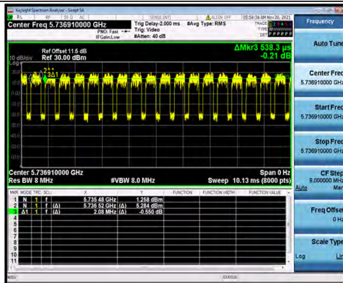
11AX20MIMO_Ant2_5745_26Tone_RU4
