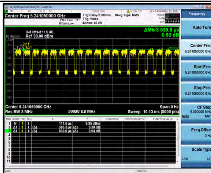
11AX20MIMO_Ant1_5240_26Tone_RU4
