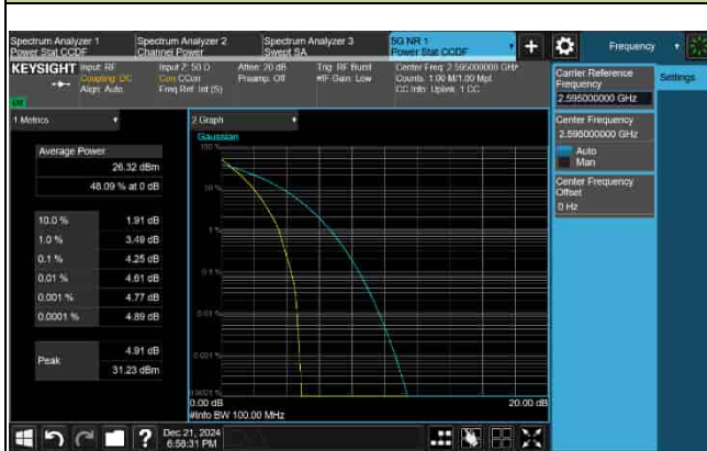
PAPR_5G_n41_30KHz_90M_2595MHz-16QAM
