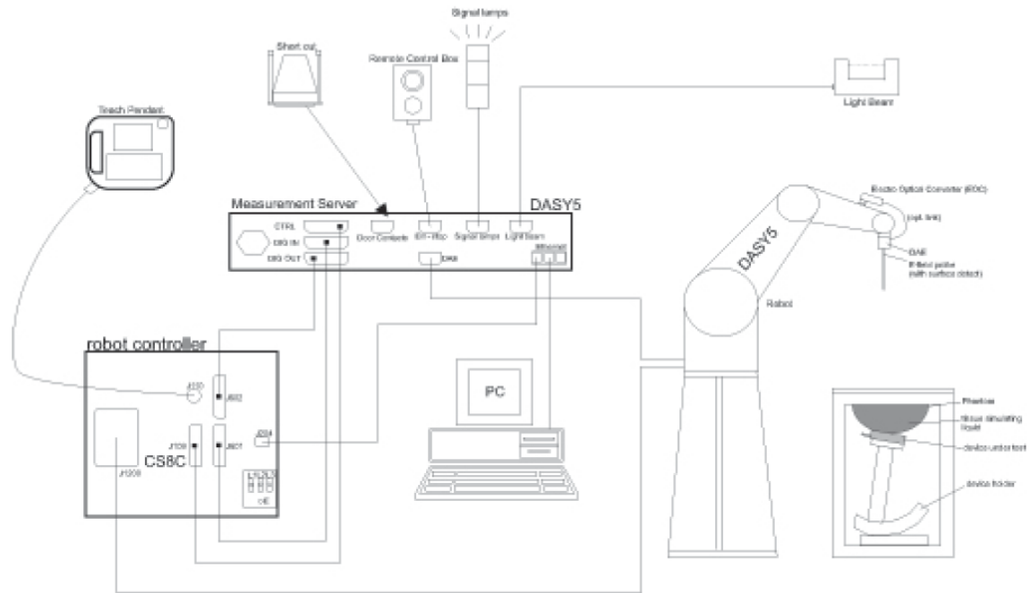
Fig. 5.1 DASY5 System
