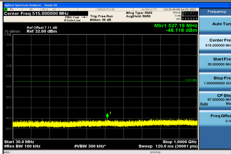
Band2-3MHz-QPSK-19185-1RB#0-30~1000MHz
