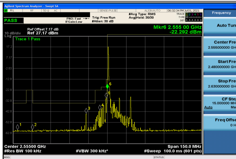
Band41-10MHz-QPSK-40290-1RB#0
