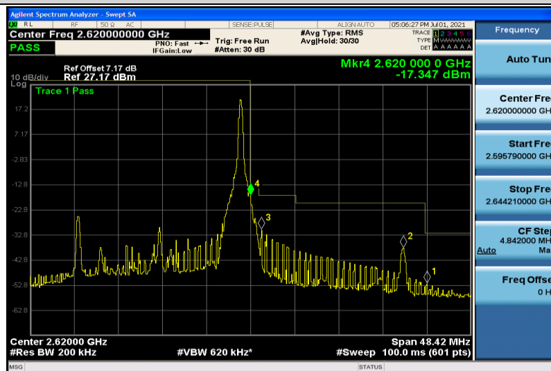
Band38-20MHz-QPSK-38150-1RB#99
