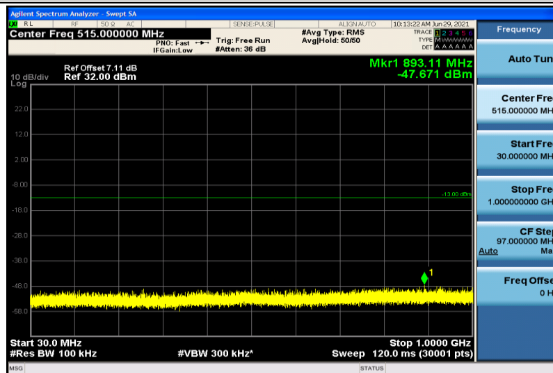
Band2-3MHz-QPSK-18615-1RB#0-30~1000MHz
