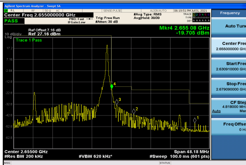
Band41-20MHz-QPSK-41140-1RB#99
