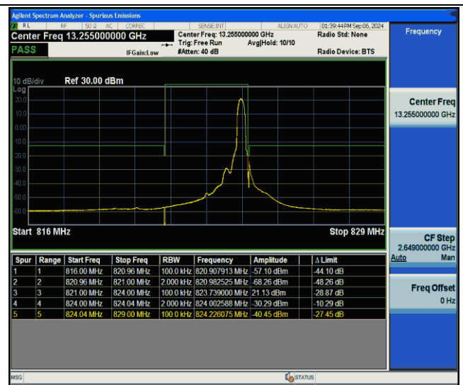
26(814-824)-3MHz-QPSK-26775-1RB#14-PASS
