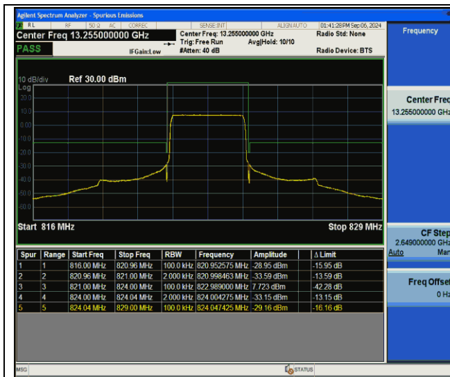
26(814-824)-3MHz-QPSK-26775-15RB#0-PASS
