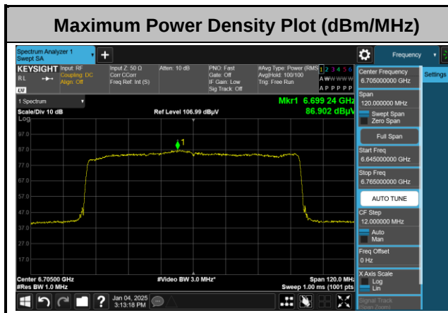
&lt;802.11be EHT80&gt;
