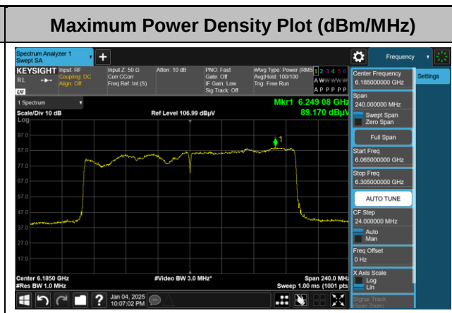
&lt;802.11be EHT160&gt;
