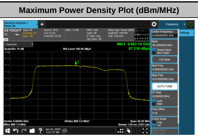
&lt;802.11be EHT40&gt;
