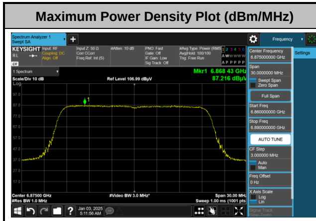
&lt;802.11be EHT20&gt;
