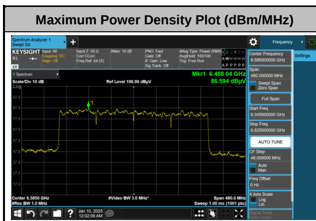
&lt;802.11be EHT320&gt;
