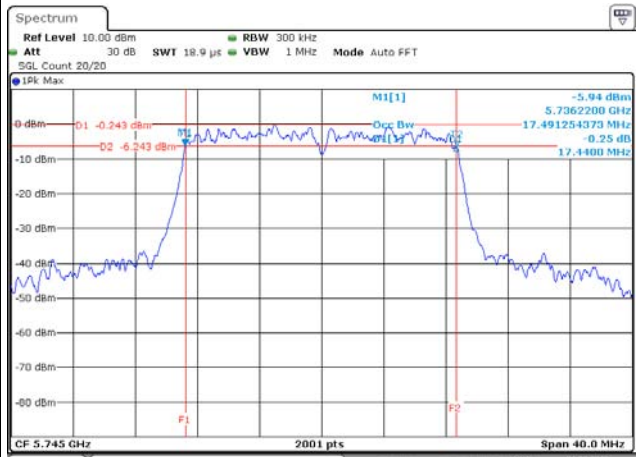
11N5.8G-20M – F1 [Port 1]
