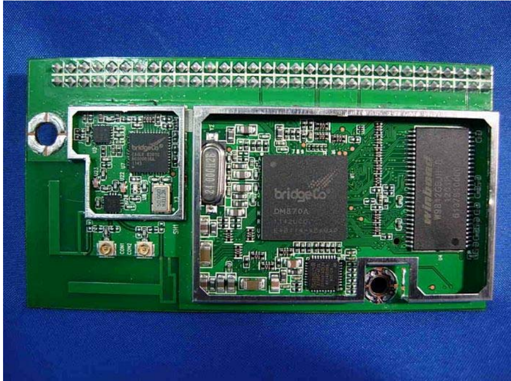
(23) EUT Photo (RF Module)
