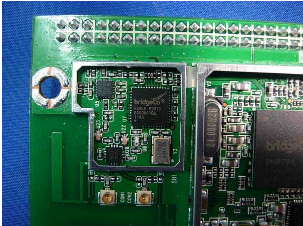
(24) EUT Photo (RF Module)
