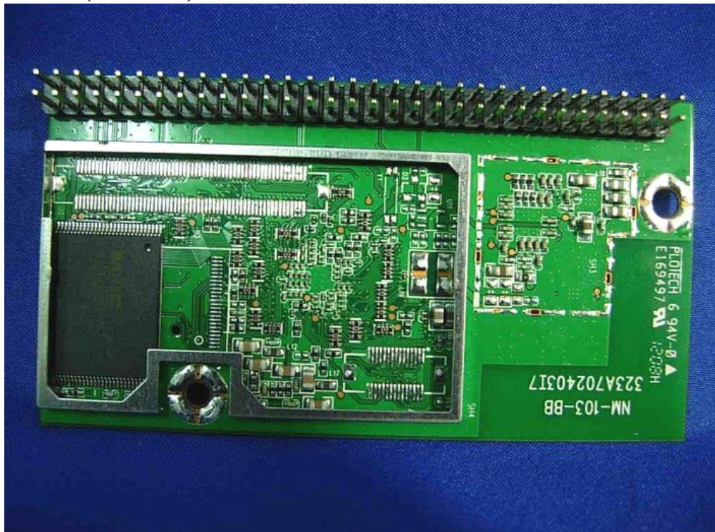
(26) EUT Photo (RF Module)
