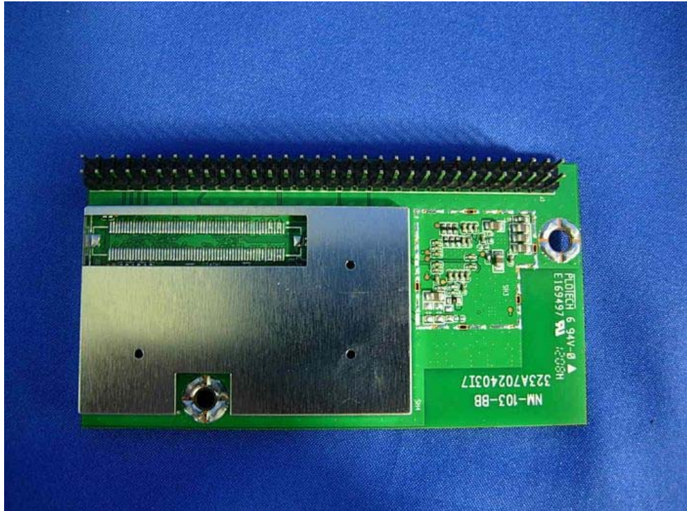
(21) EUT Photo (RF Module)
