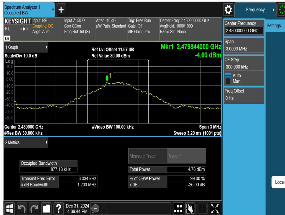
DH5-Ant1-2480
