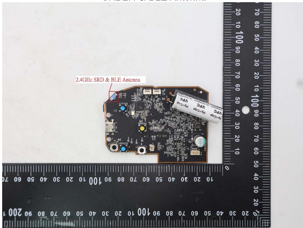
SRD2.4 & BLE Antenna
