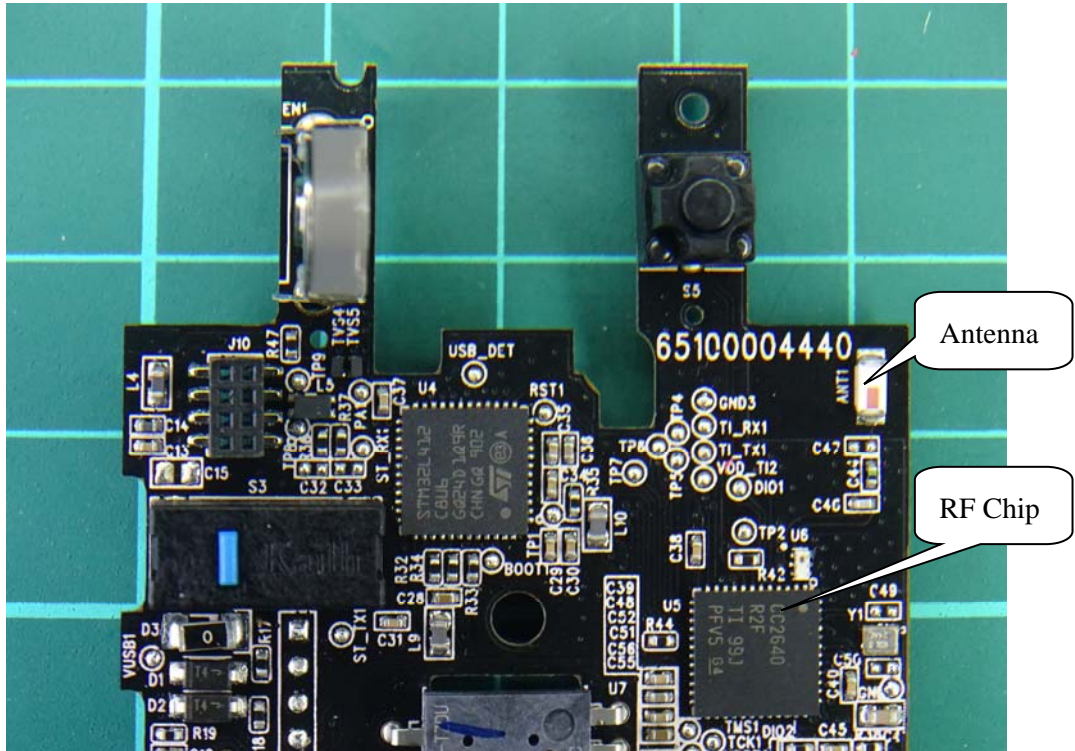
(16) EUT Photo
