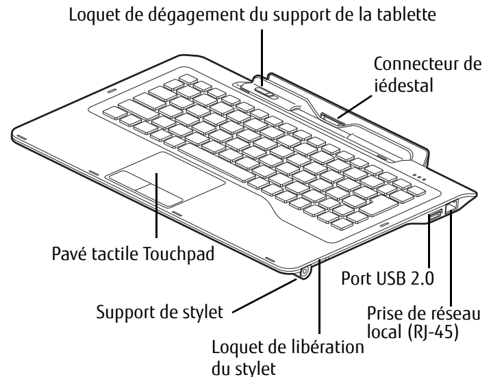
Figure 23. Station d'arrimage - avant
