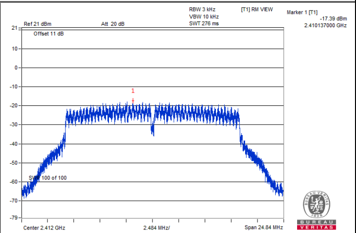
802.11g : CH 1
