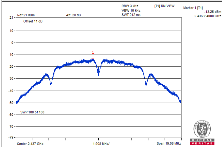
802.11b : CH 6
