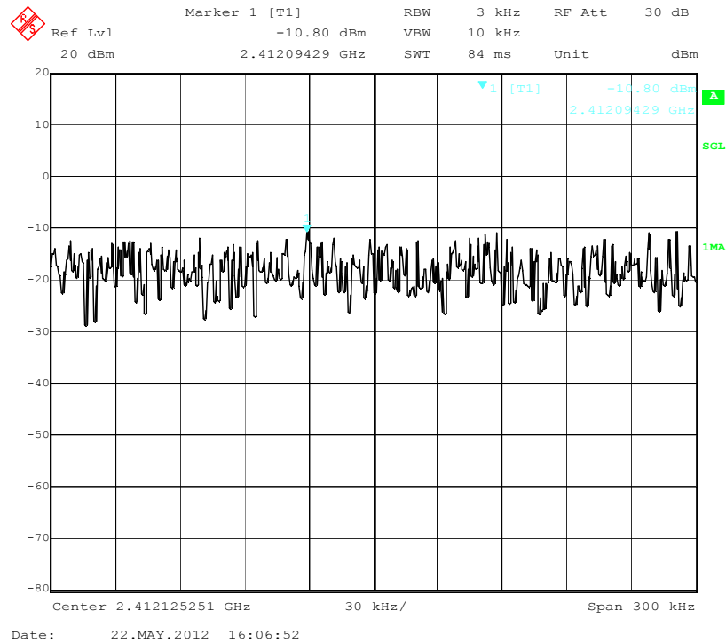
PSD Low Channel( 802.11b)
