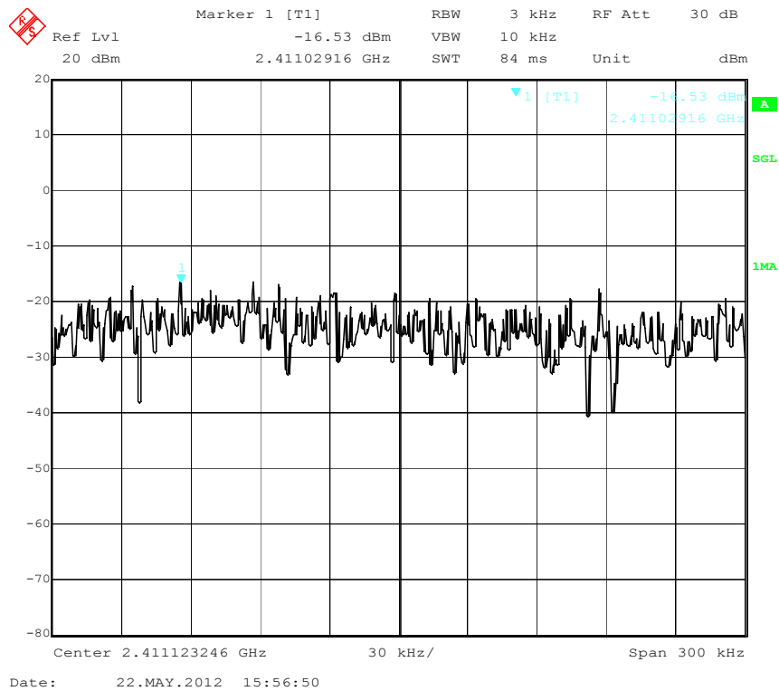
PSD Low Channel( 802.11n-20MHz-2.4G)
