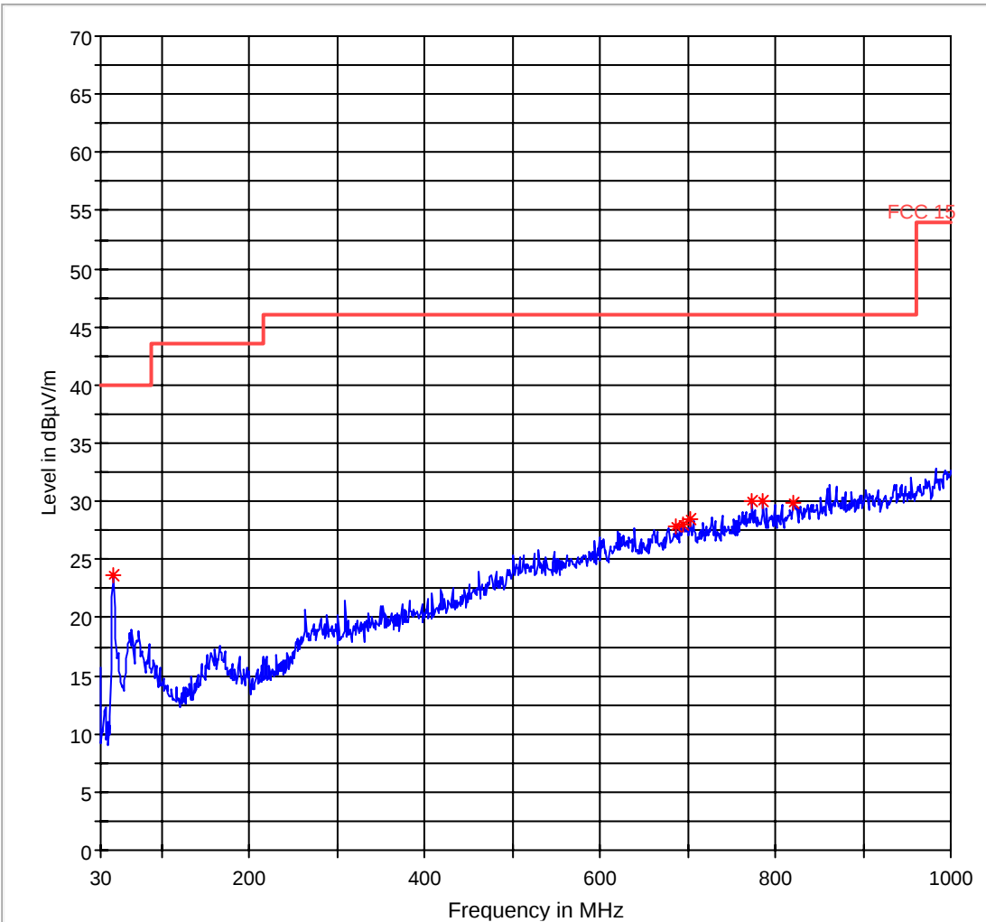
FCC 15 30-1000MHz
