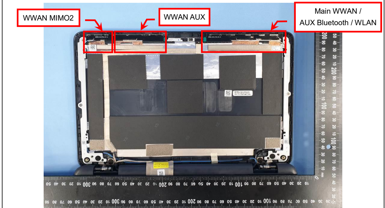
EUT Photo (44)
