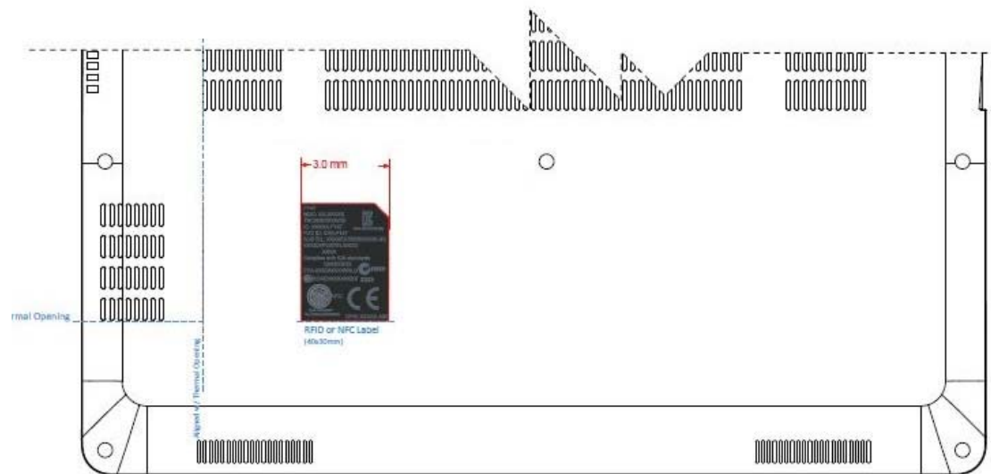
P26S BOTTOM DOOR
