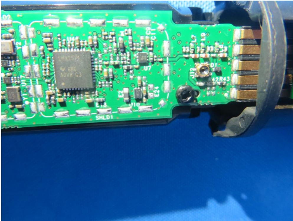
(7) EUT Photo (SLXD2 J52)
