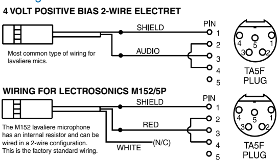
Fig. 3 - DPA Microphones
