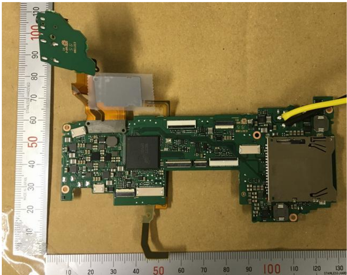
WB MAIN_B
