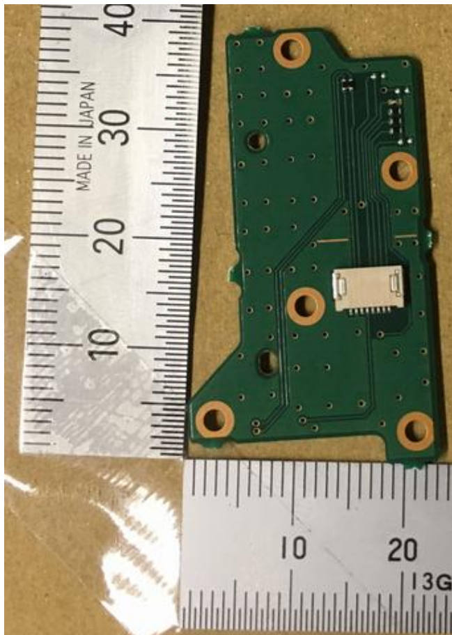
PWB REAR_B
