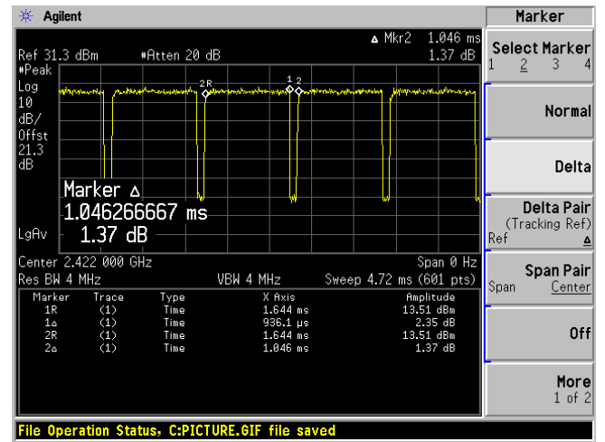
802.11n40 mode
