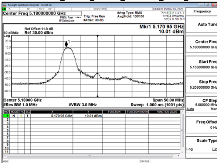
802.11ax_20MHz_ChainA_5180MHz_RU26_0
