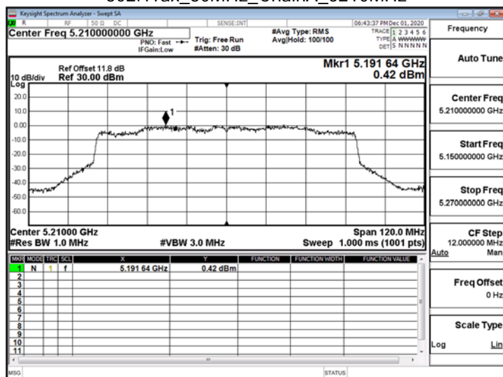
802.11ax_80MHz_ChainA_5210MHz_RU484_65
