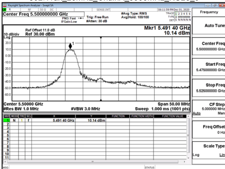
802.11ax_20MHz_ChainA_5500MHz_RU26_0
