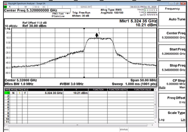
802.11ax_20MHz_ChainA_5320MHz_RU26_8
