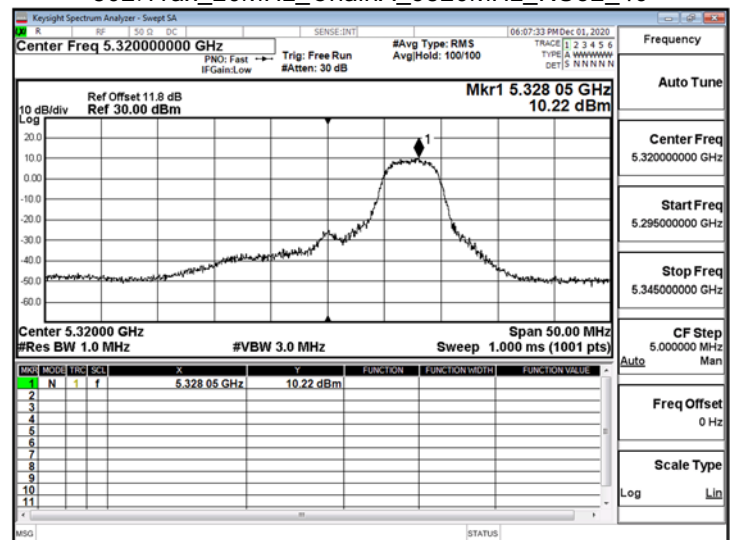
802.11ax_20MHz_ChainA_5320MHz_RU52_40
