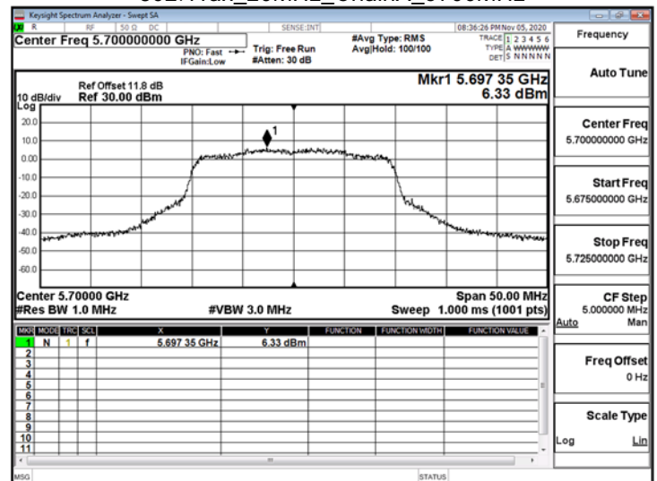
802.11ax_20MHz_ChainA_5700MHz
