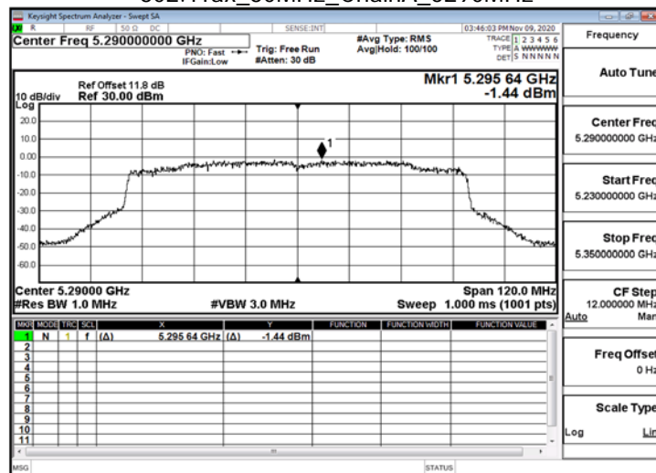
802.11ax_80MHz_ChainA_5290MHz_RU484_66
