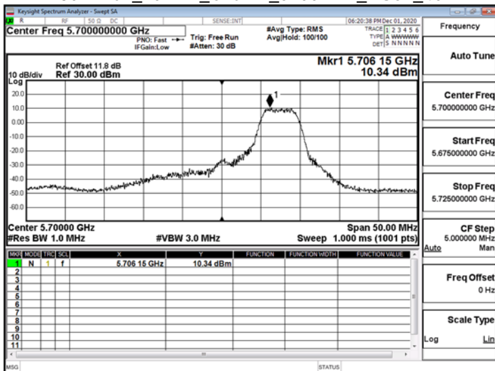
802.11ax_20MHz_ChainA_5700MHz_RU52_40
