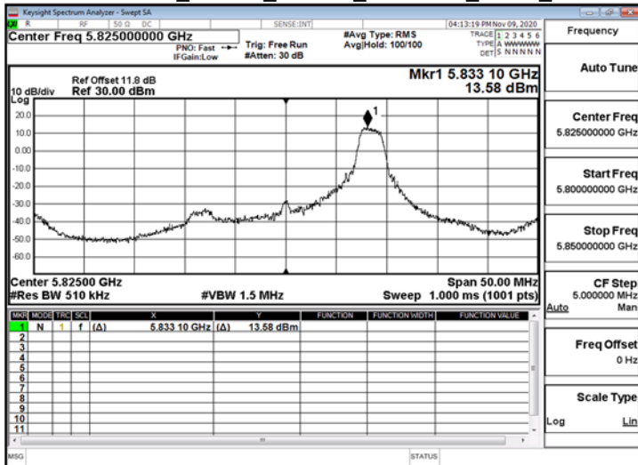
802.11ax_20MHz_ChainA_5825MHz_RU52_40
