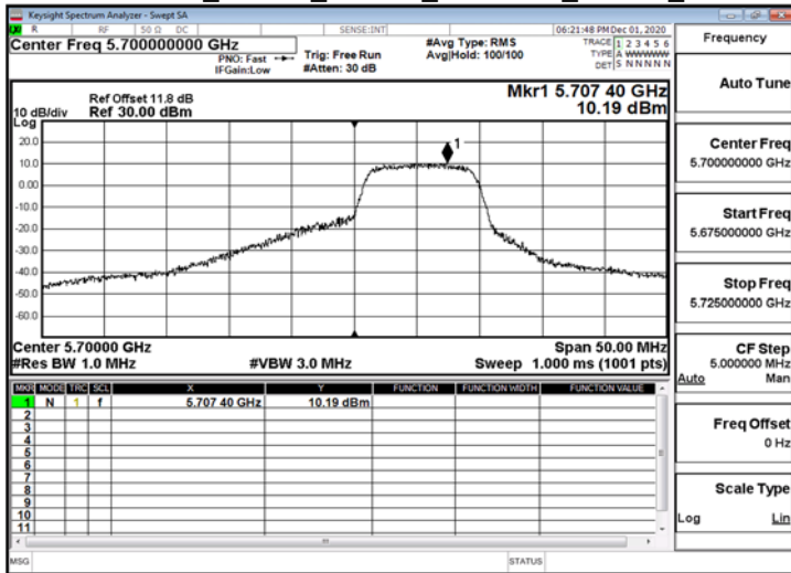
802.11ax_20MHz_ChainA_5700MHz_RU26_8
