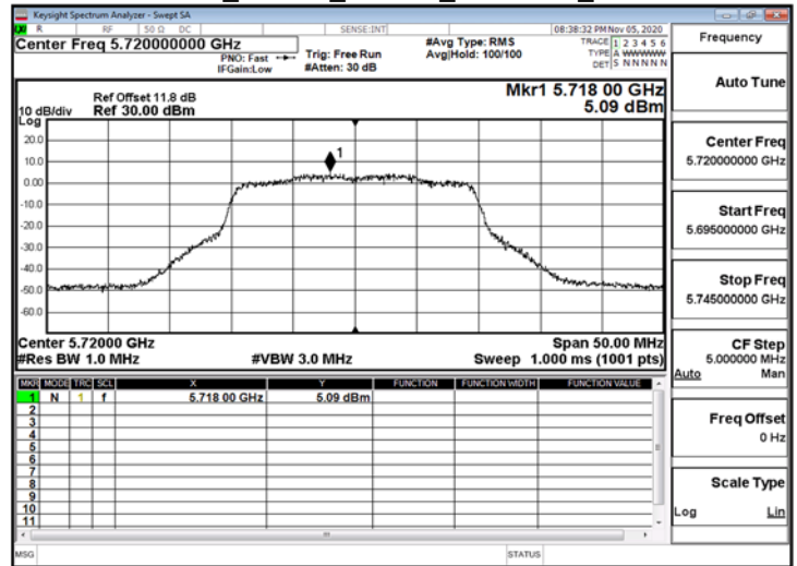
802.11ax_20MHz_ChainA_5720MHz_UNII 3
