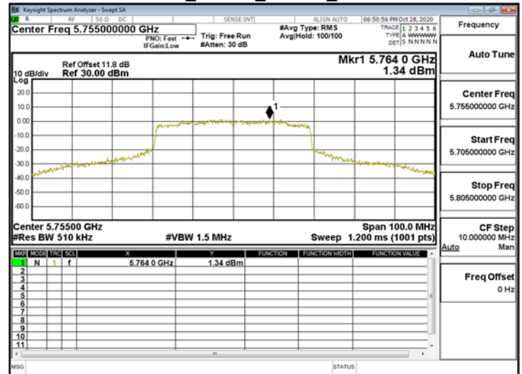
802.11ax_40MHz_ChainA_5755MHz_RU242_61
