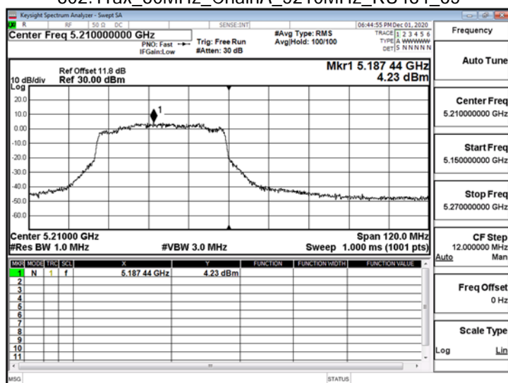
802.11ax_80MHz_ChainA_5210MHz_RU484_65
