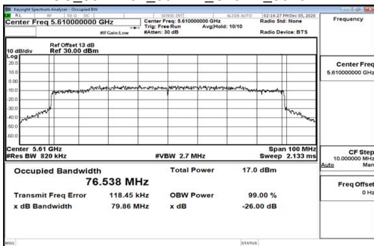
FCC_802.11ax_80MHz_Chain1_5610MHz
