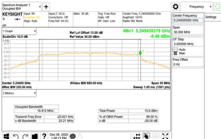
FCC_802.11ax_20MHz_Chain1_5240MHz
