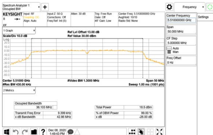
FCC_802.11n_40MHz_Chain0_5510MHz
