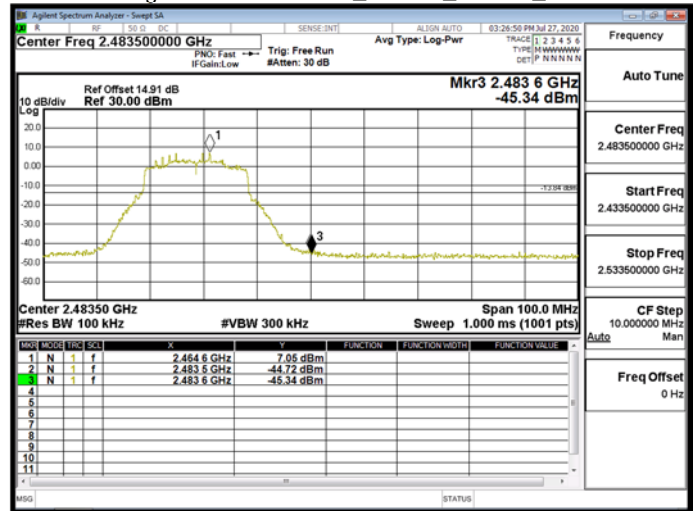
Band Edge\WLAN\802.11ax_20MHz_Chain1_2462MHz
