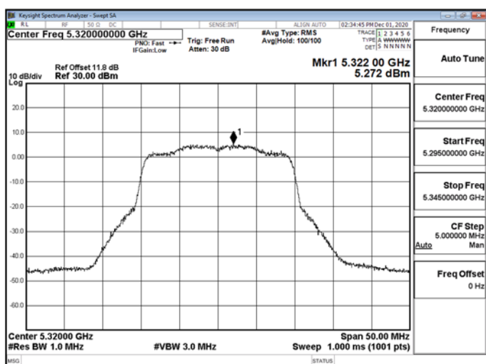
802.11ax_20MHz_5320MHz-5320
