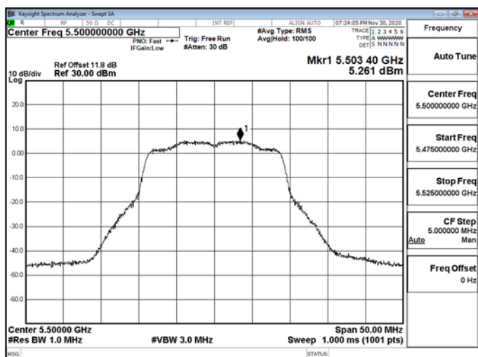
802.11n_20MHz_5500MHz-5500
