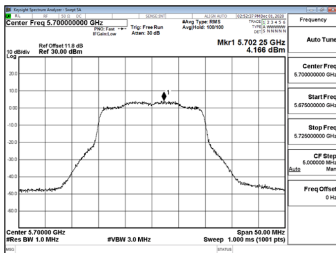
802.11ax_20MHz_5700MHz-5700
