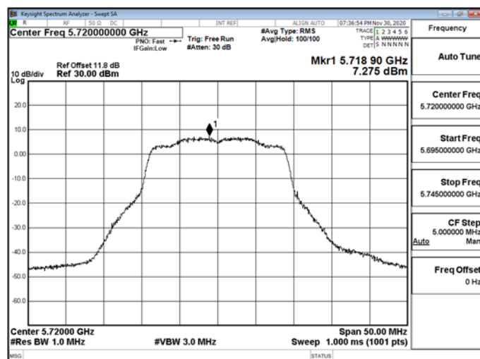
802.11n_20MHz_5720MHz_UNII 2C
