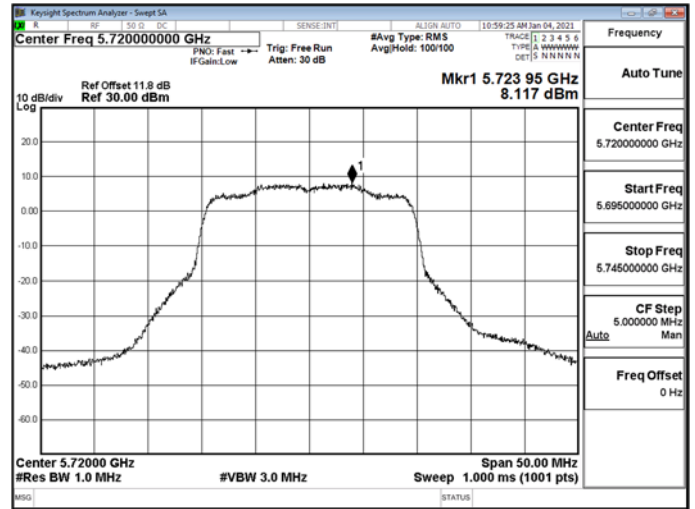
802.11ax_20MHz_5720MHz_UNII 3
