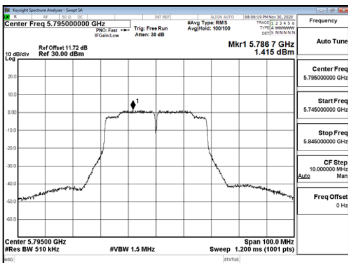
802.11n_40MHz_5795MHz-5795
