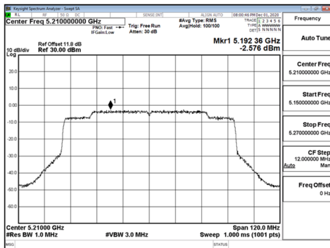
802.11ax_80MHz_RU_484_65_5210MHz-5210
