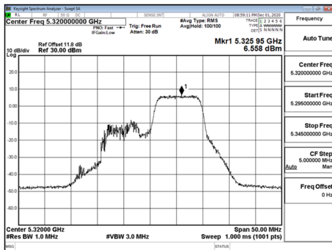
802.11ax_20MHz_RU_26_8_5320MHz-5320
