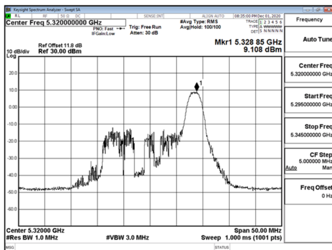
802.11ax_20MHz_RU_52_40_5320MHz-5320
