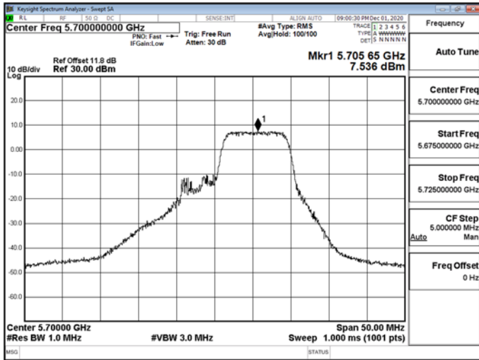
802.11ax_20MHz_RU_26_8_5700MHz-5700
