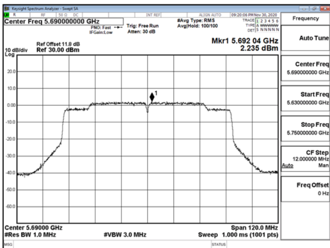
802.11ac_80MHz_5690MHz_UNII 3
