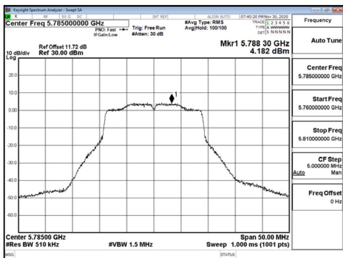
802.11n_20MHz_5785MHz-5785
