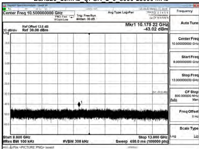
Band26 10MHz QPSK 1 0 8000-13000 MHz
