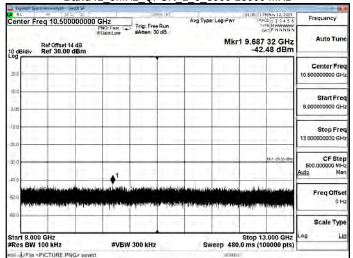
Band41 5MHz QPSK 1 0 8000-13000 MHz
