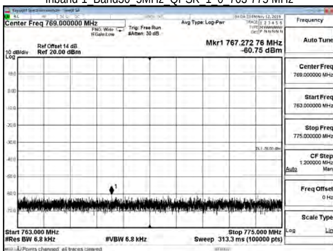
Inband-1 Band30 5MHz QPSK 1 0 763-775 MHz
