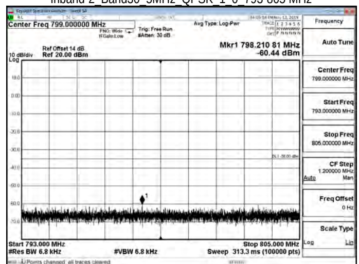
Inband-2 Band30 5MHz QPSK 1 0 793-805 MHz
