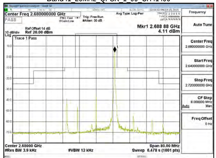
Band41 20MHz QPSK 1 99 CH41490
