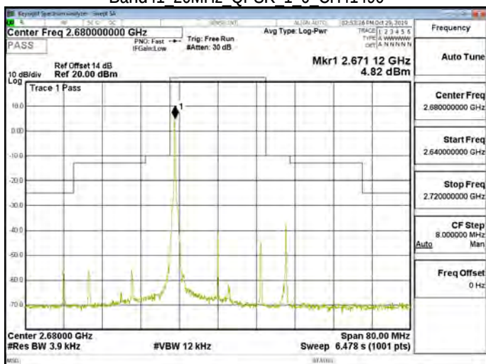
Band41 20MHz QPSK 1 0 CH41490
