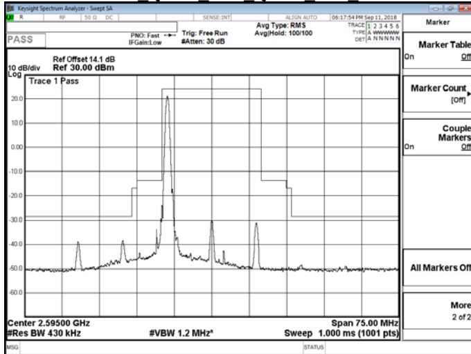
Band 38 QPSK 20M QPSK MID RB1,99
