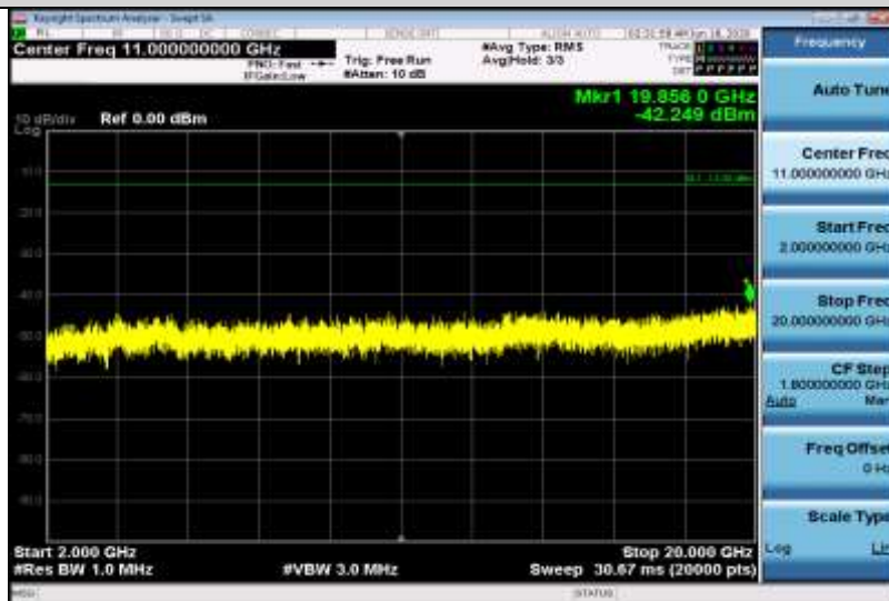
Band2-3MHz-QPSK-18900-1RB#0-Range3:2000~20000MHz
