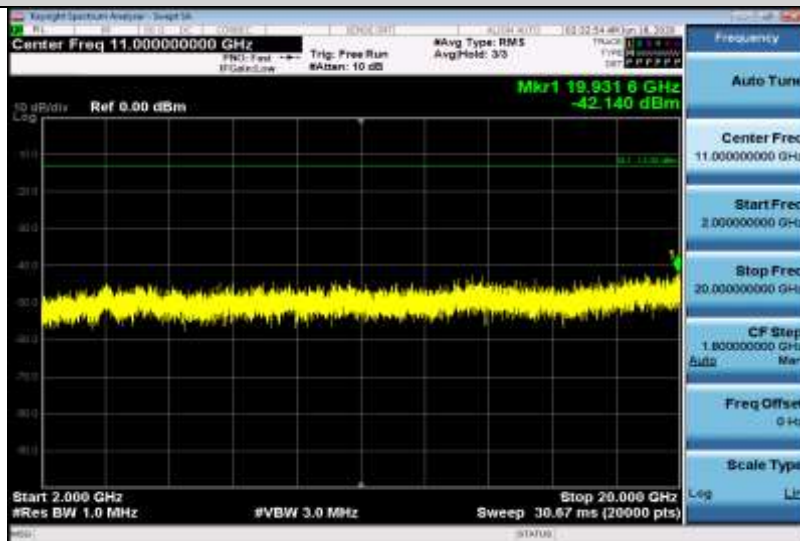
Band2-3MHz-QPSK-19185-1RB#0-Range3:2000~20000MHz
