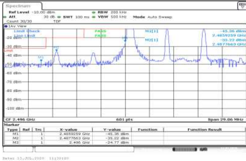
Band41-10MHz-QPSK-39700-50RB#0
