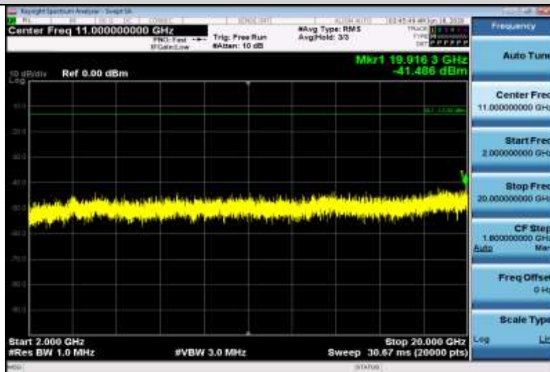
Band2-20MHz-QPSK-18900-1RB#0-Range3:2000~20000MHz
