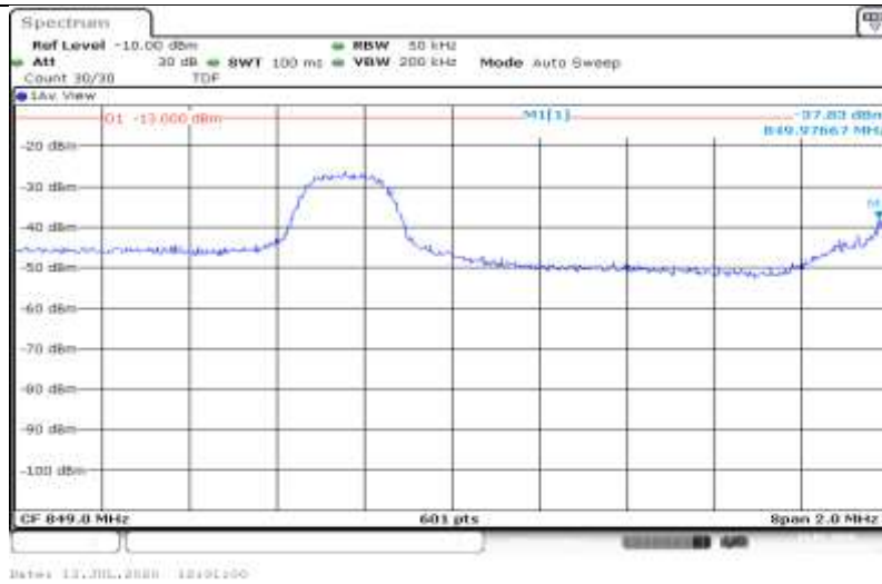
Band5-3MHz-QPSK-20635-1RB#14
