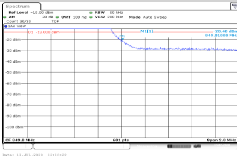
Band5-3MHz-QPSK-20635-15RB#0
