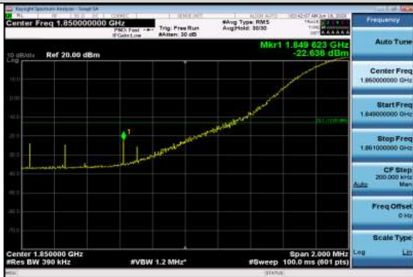
Band2-20MHz-16QAM-18700-1RB#0
