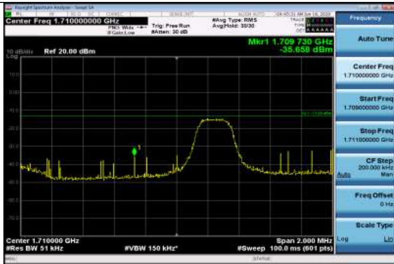
Band4-3MHz-QPSK-19965-1RB#0
