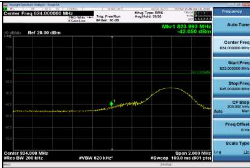
Band5-10MHz-QPSK-20450-1RB#0
