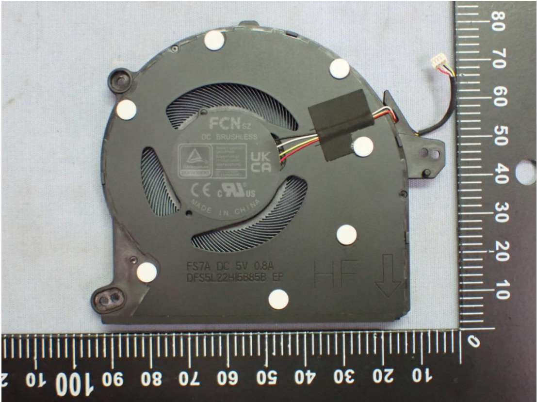
Figure 49 DC Fan
