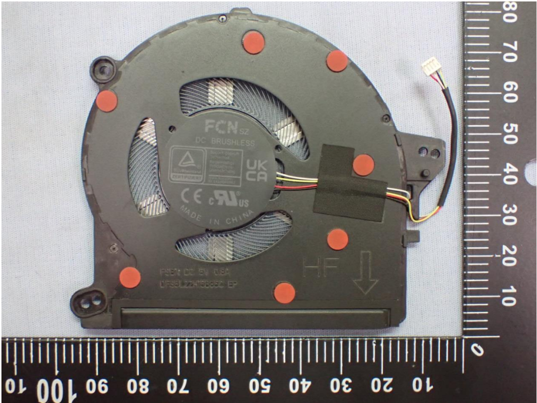
Figure 48 DC Fan
