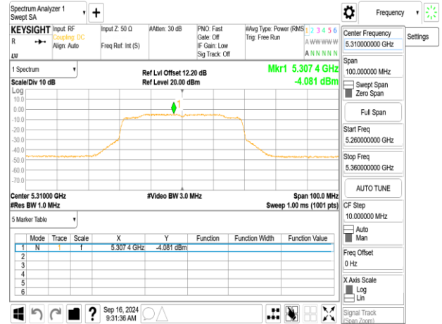
802.11be_40MHz_ChainB_5310MHz_RU242_62
