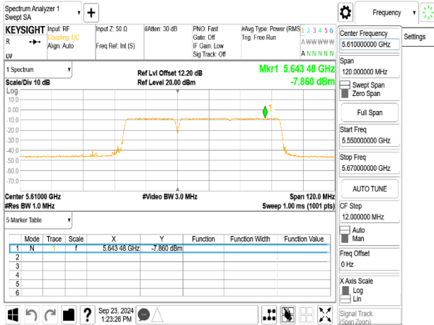
802.11be_80MHz_ChainA_5610MHz_RU484_66
