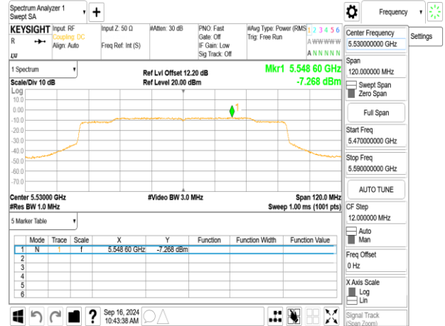
802.11be_80MHz_ChainB_5530MHz_484+242_MRU4
