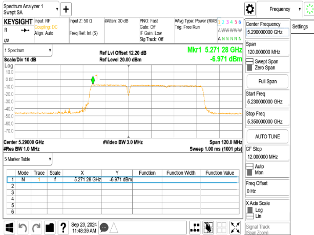
802.11be_80MHz_ChainA_5290MHz_RU484_66
