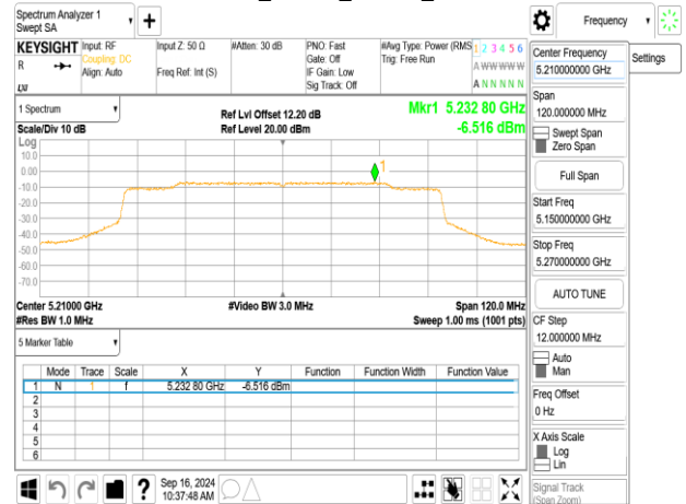
802.11be_80MHz_ChainB_5210MHz_484+242_MRUI4
