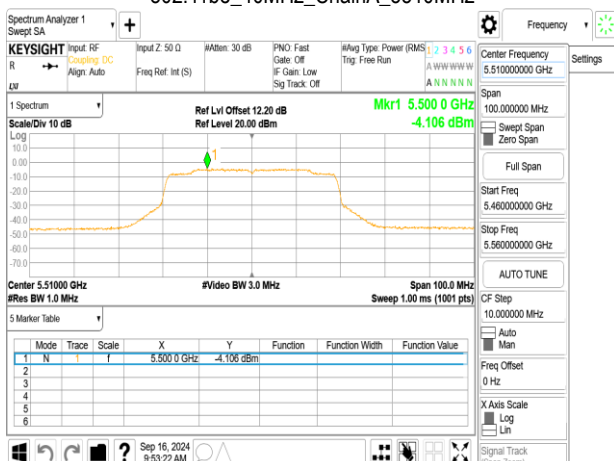
802.11be_40MHz_ChainA_5510MHz
