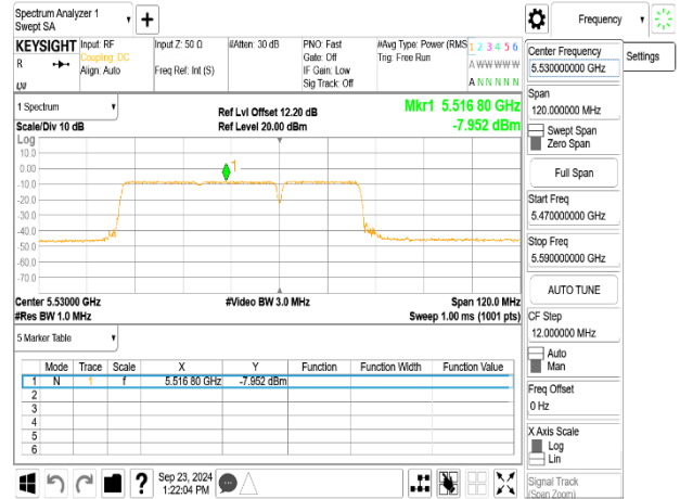
802.11be_80MHz_ChainA_5530MHz_RU484_65
