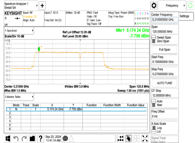
802.11be_80MHz_ChainA_5210MHz_RU484_65
