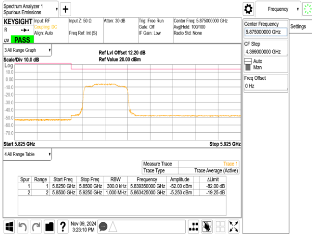
802.11be_40MHz_ChainB_5875MHz_RU242_62
