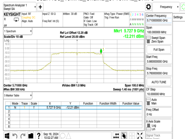
802.11be_40MHz_ChainB_5710MHz_UNII 3
