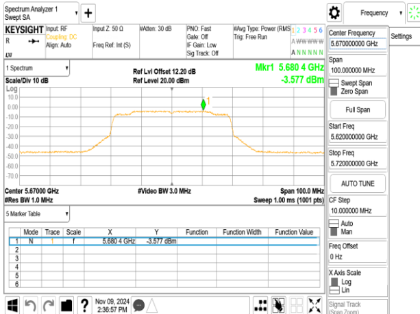
802.11ax_40MHz_ChainB_5670MHz
