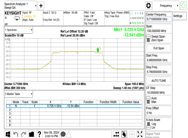
802.11ax_40MHz_ChainB_5710MHz_UNII 3
