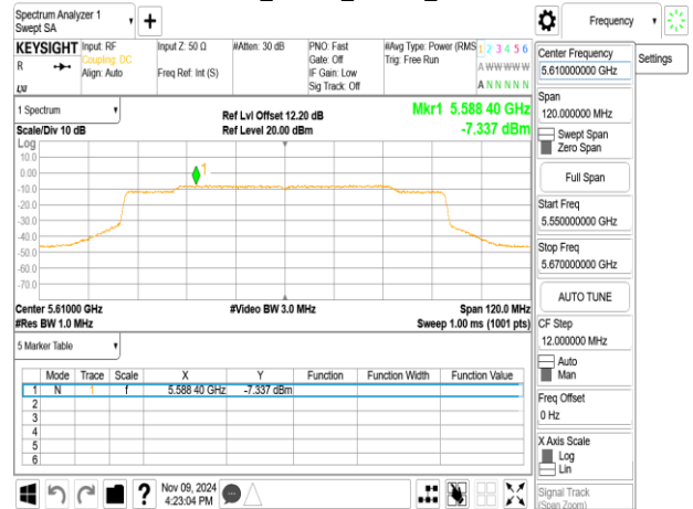
802.11ax_80MHz_ChainB_5610MHz_RU484_66
