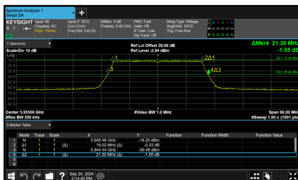
Figure 83 - 802.11ax HE20 SU LPI Minimum 99% OBW
