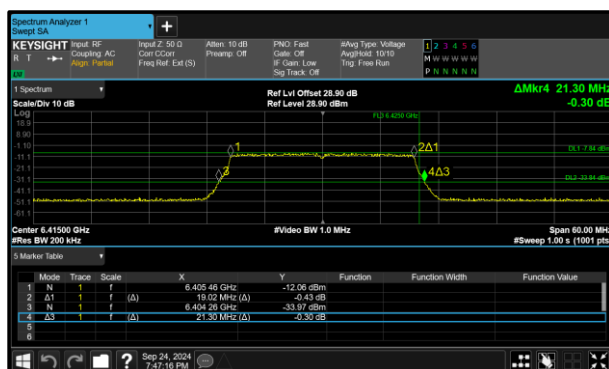
Figure 129 - 802.11ax HE20 SU LPI Minimum 99% OBW
