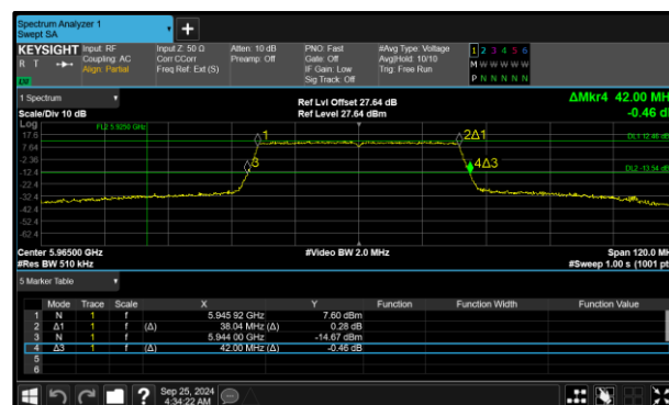
Figure 148 - 802.11ax HE40 SU SP Maximum 99% OBW
