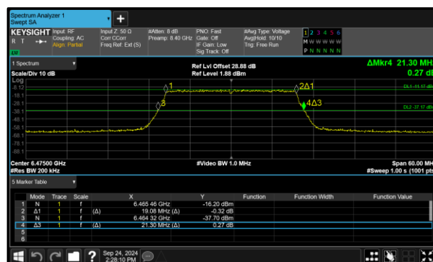
Figure 84 - 802.11ax HE20 SU LPI Maximum 99% OBW
