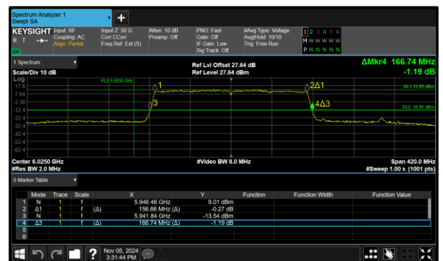
Figure 152 - 802.11ax HE160 SU SP Maximum 99% OBW
