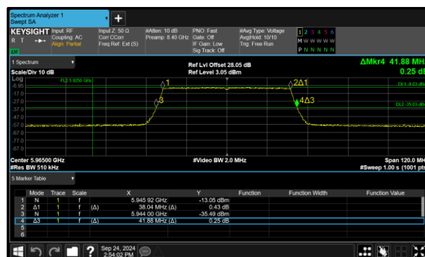
Figure 86 - 802.11ax HE40 SU LPI Maximum 99% OBW
