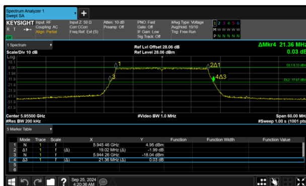
Figure 145 - 802.11ax HE20 SU SP Minimum 99% OBW
