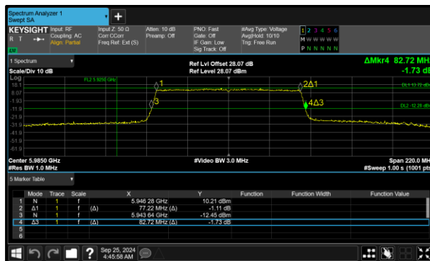
Figure 149 - 802.11ax HE80 SU SP Minimum 99% OBW
