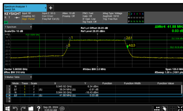
Figure 100 - 802.11ax HE40 SU SP Maximum 99% OBW
