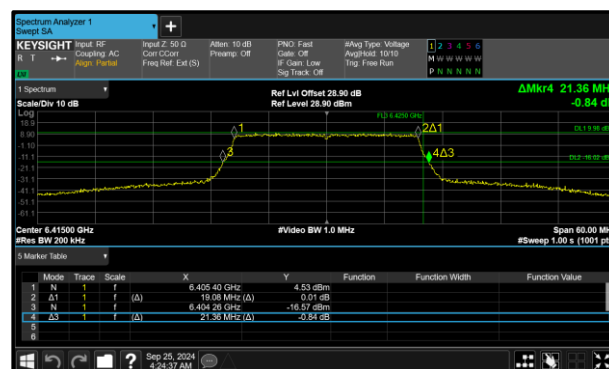
Figure 146 - 802.11ax HE20 SU SP Maximum 99% OBW
