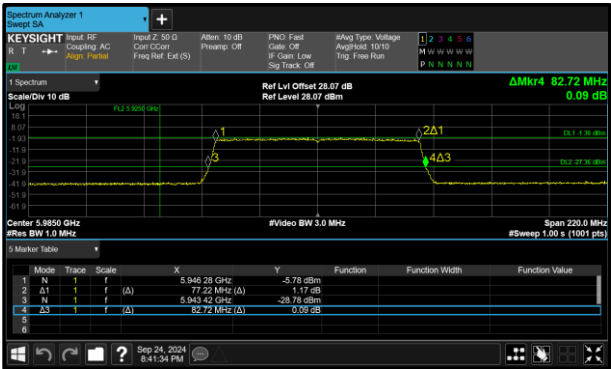
Figure 133 - 802.11ax HE80 SU LPI Minimum 99% OBW
