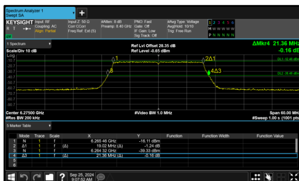
Figure 137 - 802.11ax HE20 SU VLP Minimum 99% OBW
