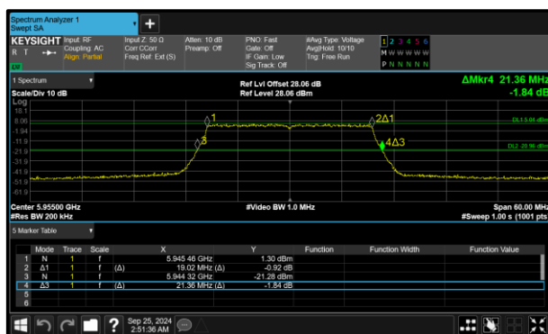
Figure 97 - 802.11ax HE20 SU SP Minimum 99% OBW
