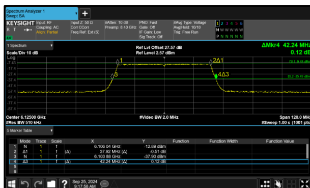
Figure 139 - 802.11ax HE40 SU VLP Minimum 99% OBW
