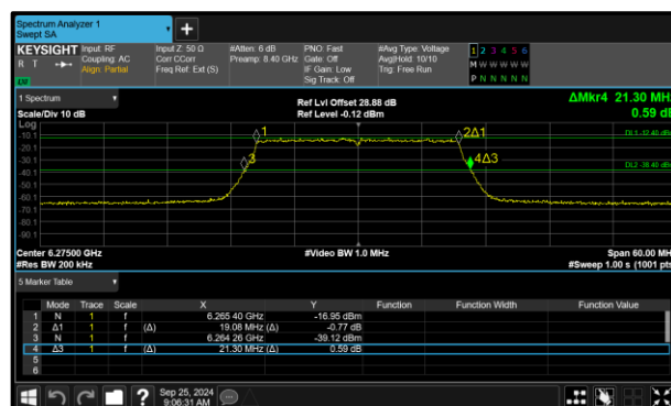
Figure 138 - 802.11ax HE20 SU VLP Maximum 99% OBW
