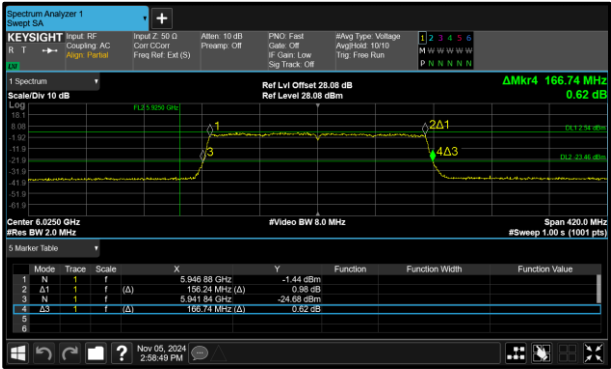
Figure 135 - 802.11ax HE160 SU LPI Minimum 99% OBW
