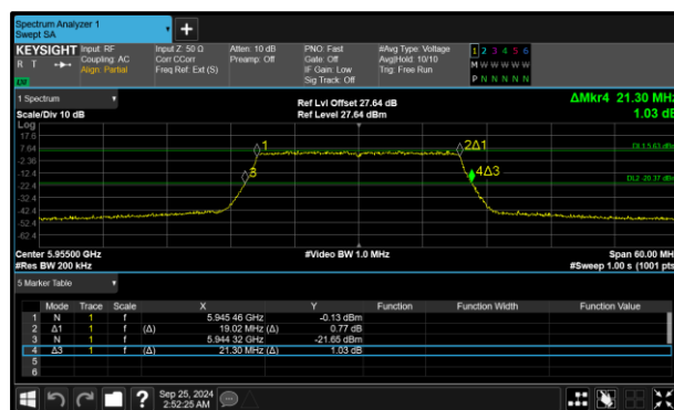
Figure 98 - 802.11ax HE20 SU SP Maximum 99% OBW
