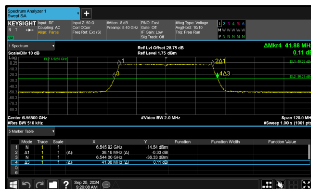
Figure 140 - 802.11ax HE40 SU VLP Maximum 99% OBW
