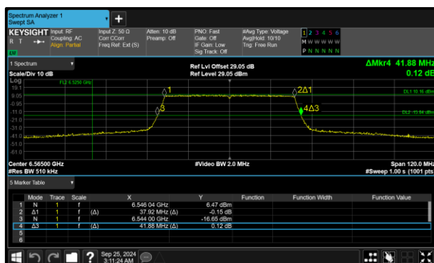
Figure 99 - 802.11ax HE40 SU SP Minimum 99% OBW
