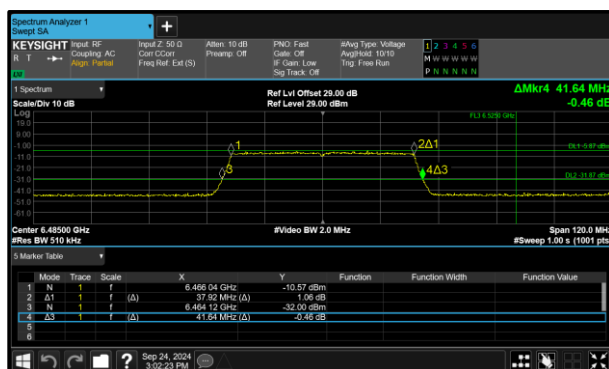
Figure 85 - 802.11ax HE40 SU LPI Minimum 99% OBW
