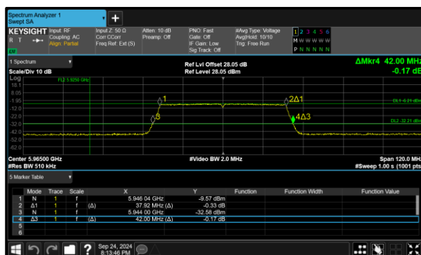
Figure 131 - 802.11ax HE40 SU LPI Minimum 99% OBW
