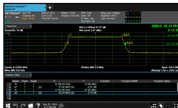
Figure 116 - 802.11ax HE40 SU VLP Maximum 26 dB EBW
