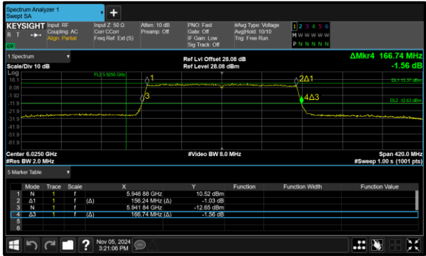
Figure 103 - 802.11ax HE160 SU SP Minimum 99% OBW
