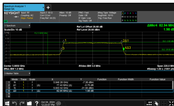
Figure 166 - 802.11ax HE80 SU LPI Maximum 99% OBW
