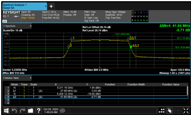
Figure 186 - 802.11ax HE40 SU Minimum 99% OBW
