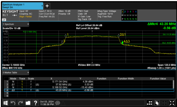
Figure 187 - 802.11ax HE40 SU Maximum 99% OBW
