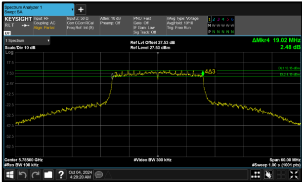
Figure 168 - 802.11ax HE20 SU Minimum 6 dB EBW
