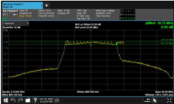
Figure 71 - 802.11ax HE20 SU Minimum 6 dB EBW
