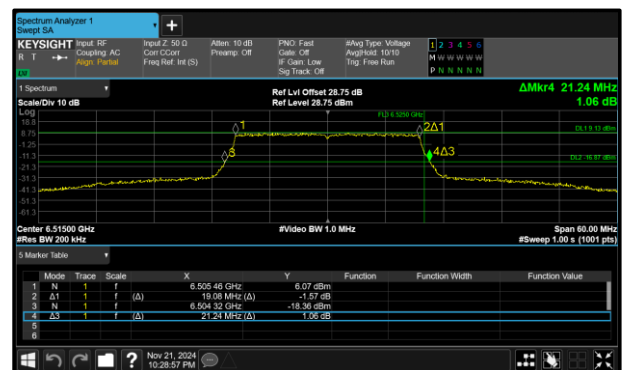
Figure 138 - 802.11ax HE20 SU SP Maximum 99% OBW
