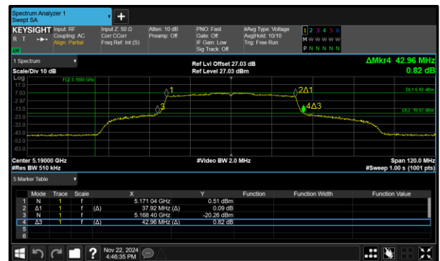
Figure 301 - 802.11ax HE40 SU Maximum 99% OBW
