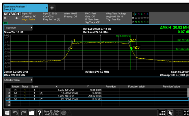
Figure 298 - 802.11ax HE20 SU Minimum 99% OBW
