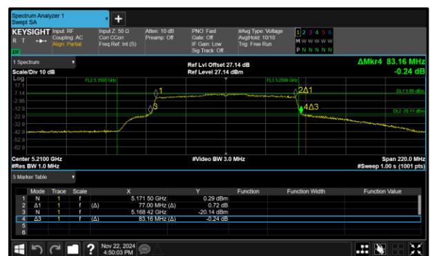
Figure 303 - 802.11ax HE80 SU Maximum 99% OBW
