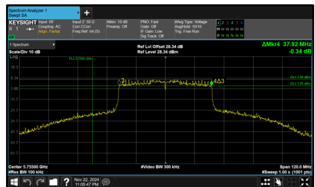
Figure 315 - 802.11ax HE40 SU Maximum 6 dB EBW
