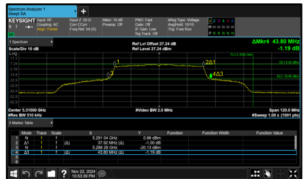
Figure 285 - 802.11ax HE40 SU Maximum 26 dB EBW
