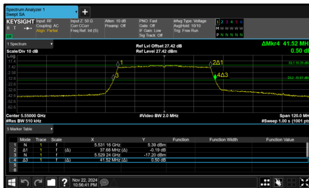
Figure 300 - 802.11ax HE40 SU Minimum 99% OBW
