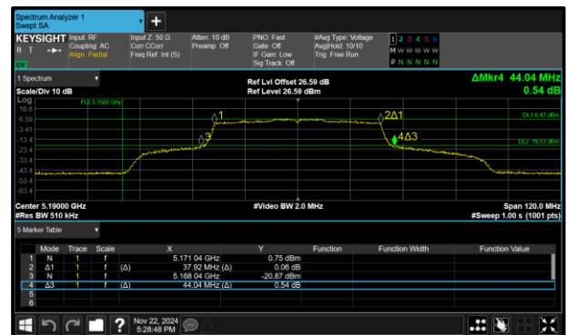
Figure 329 - 802.11ax HE40 SU Maximum 26 dB EBW
