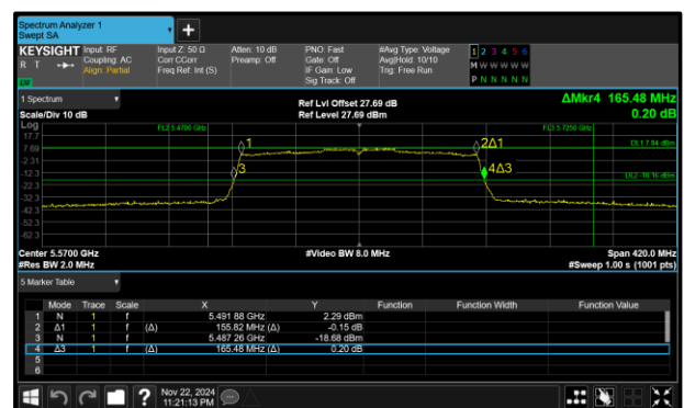
Figure 305 - 802.11ax HE160 SU Maximum 99% OBW
