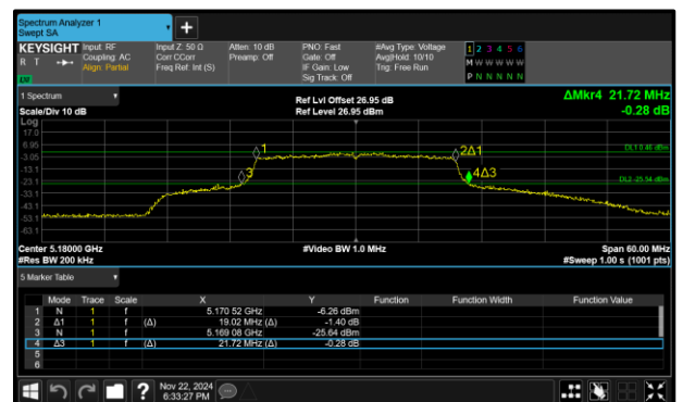
Figure 299 - 802.11ax HE20 SU Maximum 99% OBW
