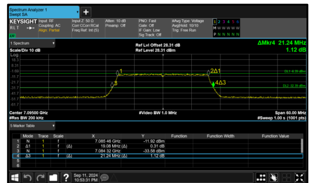
Figure 130 - 802.11ax HE20 SU LPI Maximum 99% OBW
