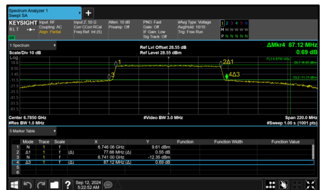
Figure 142 - 802.11ax HE80 SU SP Maximum 99% OBW
