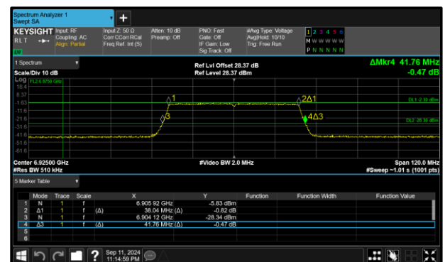
Figure 132 - 802.11ax HE40 SU LPI Maximum 99% OBW
