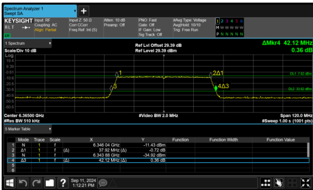
Figure 154 - 802.11ax HE40 SU LPI Maximum 26 dB EBW
