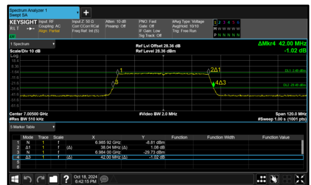
Figure 88 - 802.11ax HE40 SU LPI Maximum 99% OBW
