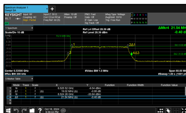
Figure 110 - 802.11ax HE20 SU LPI Maximum 26 dB EBW
