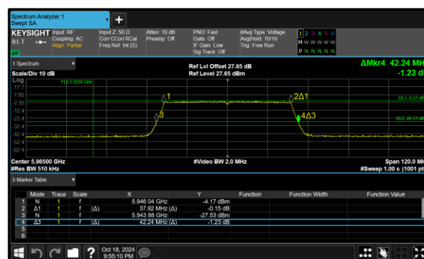
Figure 112 - 802.11ax HE40 SU LPI Maximum 26 dB EBW
