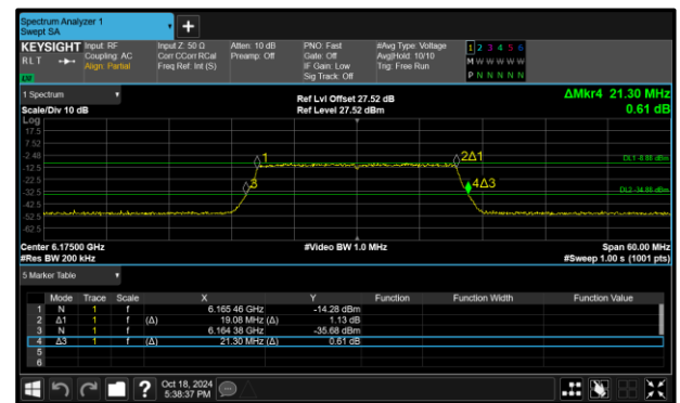
Figure 86 - 802.11ax HE20 SU LPI Maximum 99% OBW
