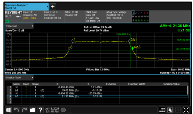
Figure 86 - 802.11ax HE20 SU SP Maximum 99% OBW
