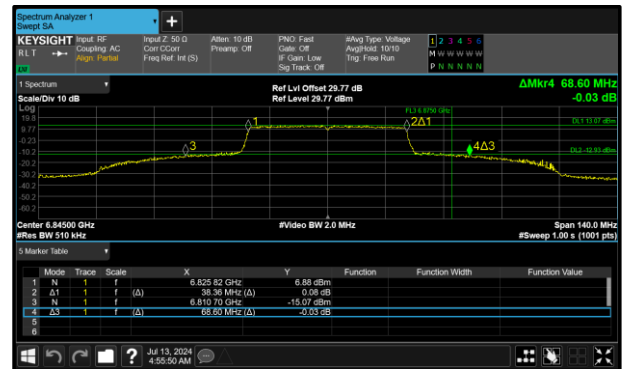
Figure 116 - 802.11ax HE40 SU SP Maximum 26 dB BW
