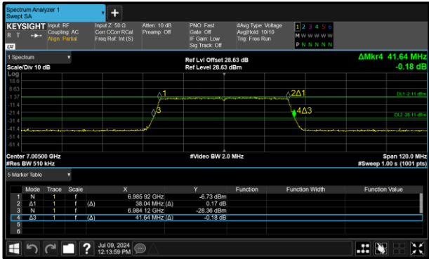
Figure 111 - 802.11ax HE40 SU LPI Minimum 26 dB EBW
