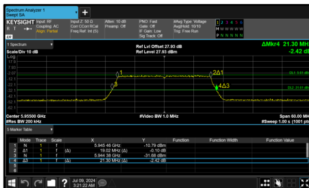
Figure 43 - 802.11ax HE20 SU LPI Minimum 99% OBW
