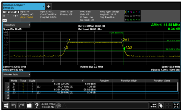
Figure 15 - 802.11ax HE40 SU LPI Minimum 26 dB EBW
