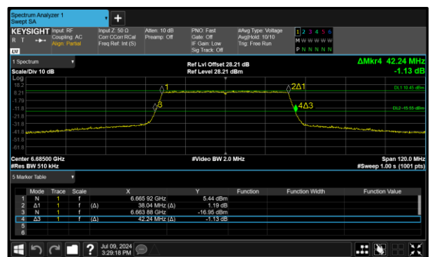
Figure 64 - 802.11ax HE40 SU SP Maximum 26 dB EBW
