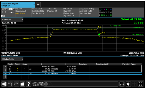
Figure 36 - 802.11ax HE40 SU SP Maximum 99% OBW
