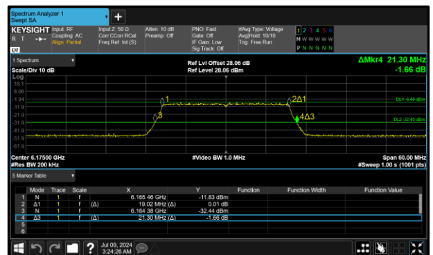
Figure 44 - 802.11ax HE20 SU LPI Maximum 99% OBW
