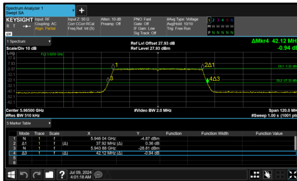
Figure 45 - 802.11ax HE40 SU LPI Minimum 99% OBW
