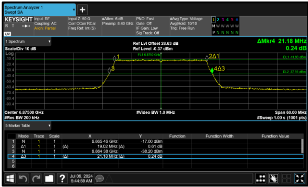
Figure 69 - 802.11ax HE20 SU LPI Minimum 26 dB EBW
