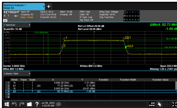
Figure 47 - 802.11ax HE80 SU LPI Minimum 99% OBW
