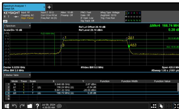
Figure 49 - 802.11ax HE160 SU LPI Minimum 99% OBW
