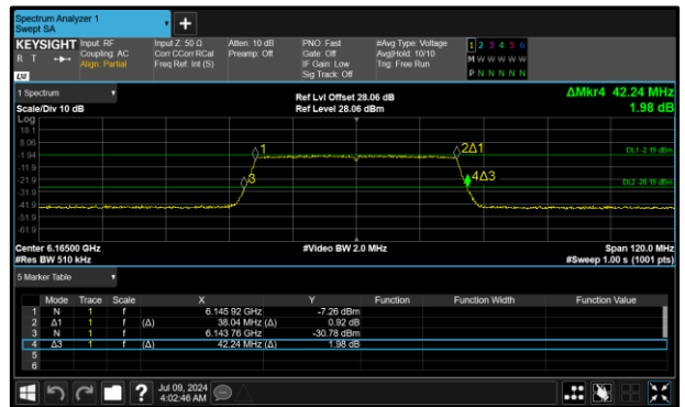
Figure 46 - 802.11ax HE40 SU LPI Maximum 99% OBW
