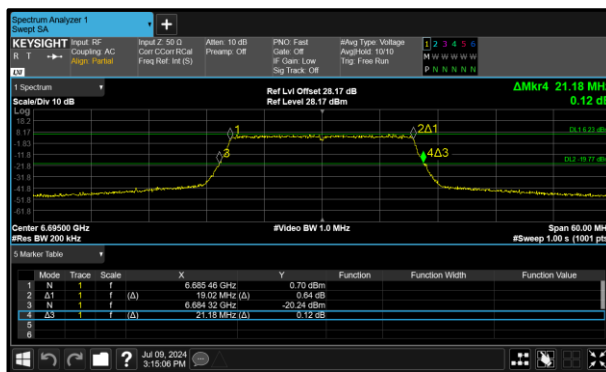
Figure 61 - 802.11ax HE20 SU SP Minimum 26 dB EBW
