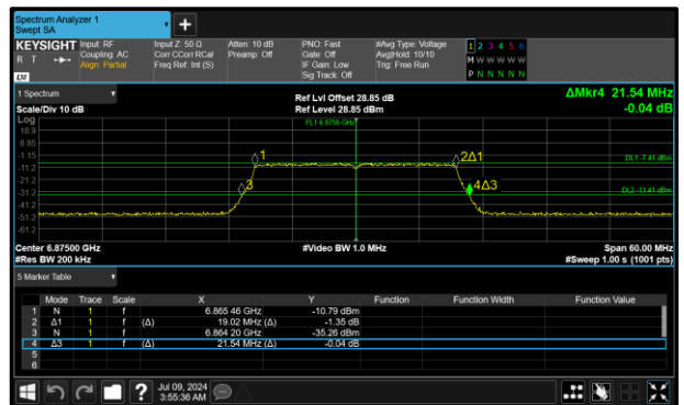
Figure 14 - 802.11ax HE20 SU LPI Maximum 26 dB EBW
