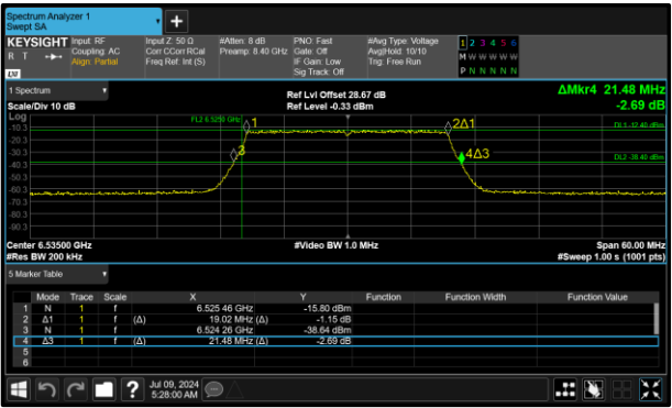
Figure 70 - 802.11ax HE20 SU LPI Maximum 26 dB EBW
