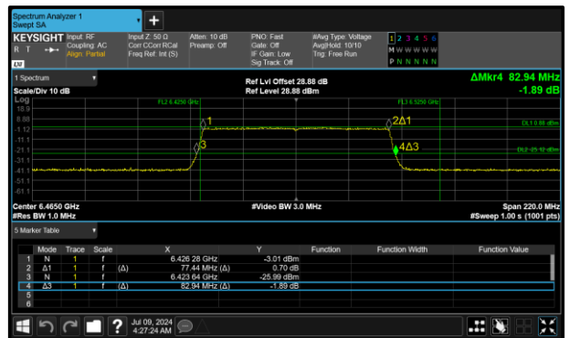
Figure 48 - 802.11ax HE80 SU LPI Maximum 99% OBW
