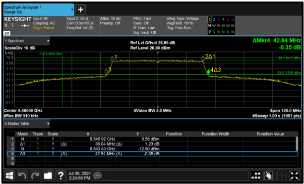
Figure 6 - 802.11ax HE40 SU SP Maximum 26 dB EBW
