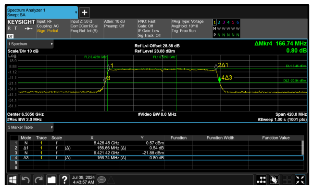
Figure 50 - 802.11ax HE160 SU LPI Maximum 99% OBW
