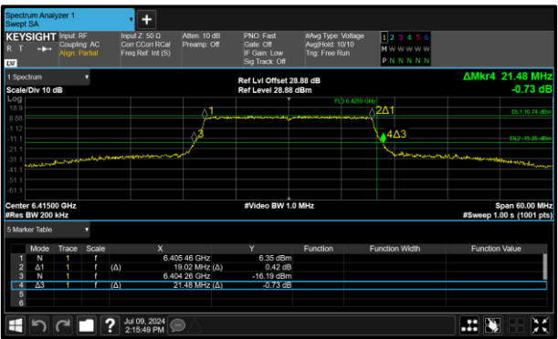
Figure 34 - 802.11ax HE20 SU SP Maximum 99% OBW
