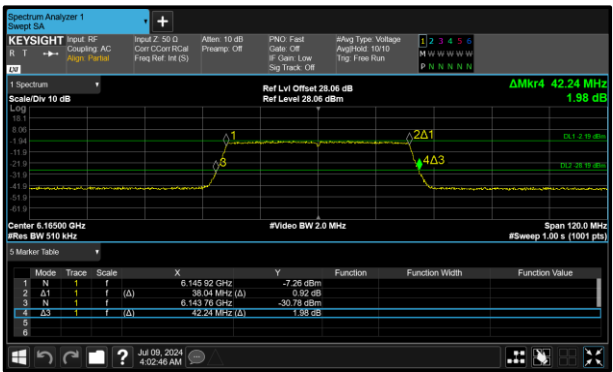
Figure 16 - 802.11ax HE40 SU LPI Maximum 26 dB EBW
