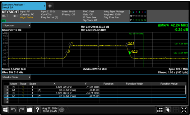
Figure 56 - 802.11ax HE40 SU VLP Maximum 99% OBW
