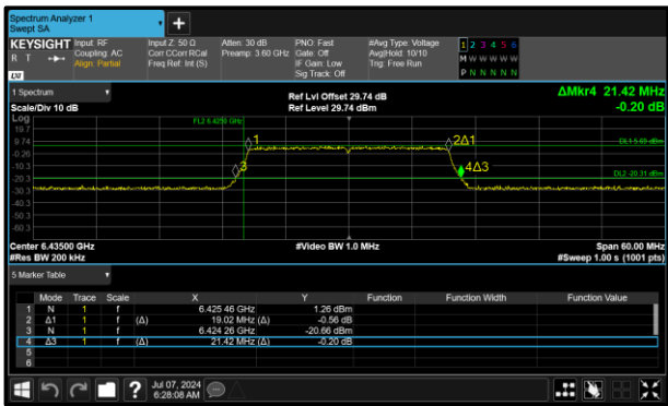
Figure 159 - 802.11ax HE20 SU SP Minimum 99% OBW
