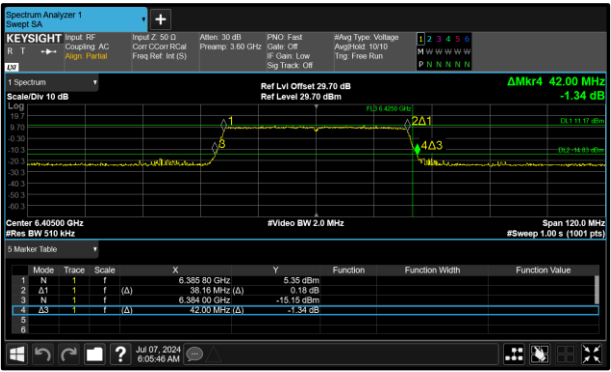
Figure 162 - 802.11ax HE40 SU SP Maximum 99% OBW
