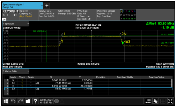
Figure 163 - 802.11ax HE80 SU SP Minimum 99% OBW
