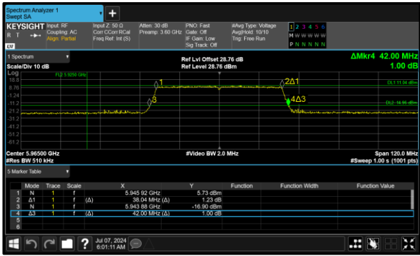
Figure 161 - 802.11ax HE40 SU SP Minimum 99% OBW
