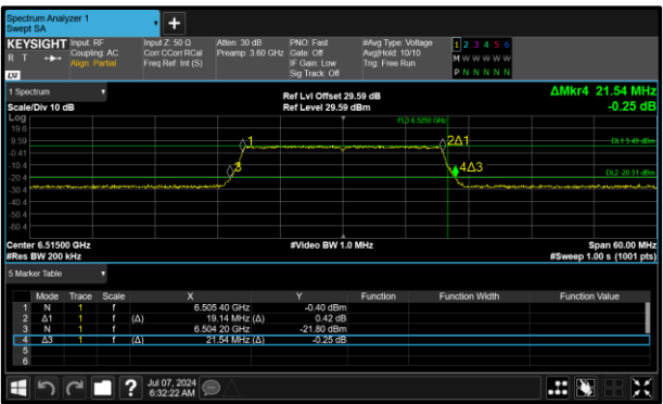
Figure 160 - 802.11ax HE20 SU SP Maximum 99% OBW
