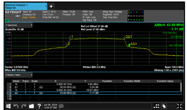
Figure 307 - 802.11ax HE40 SU Maximum 99% OBW
