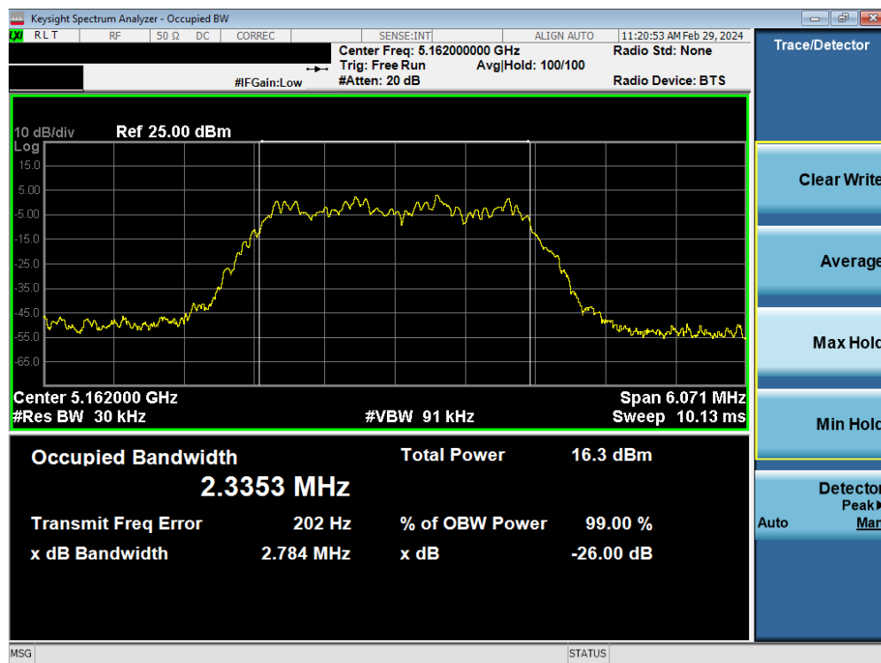
Plot 7-7. 26dB BW & 99% OBW Antenna 3a (HDR4, ePA– 5162MHz)
