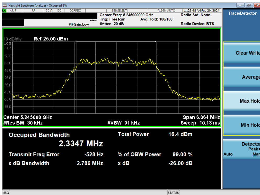
Plot 7-9. 26dB BW & 99% OBW Antenna 3a (HDR4, ePA- 5245MHz)
